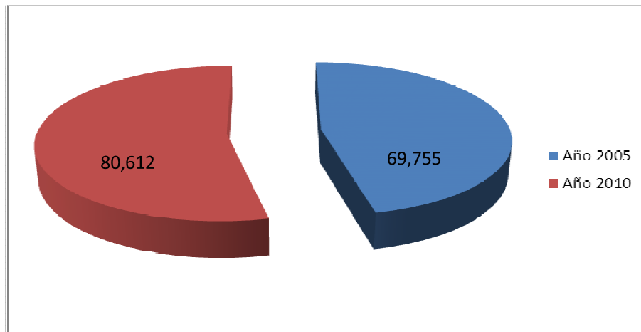
Grafica 1. Crecimiento Demográfico
