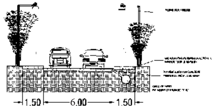
Imagen 11- Sección de camino de terracería con propuesta de equipamiento urbano
