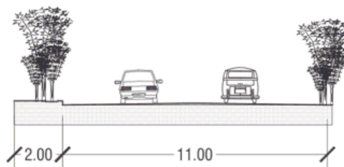
Imagen 12- Sección de vialidad principal
