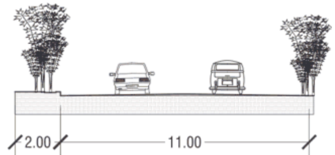
Imagen 41.- Corte de la carretera federal
