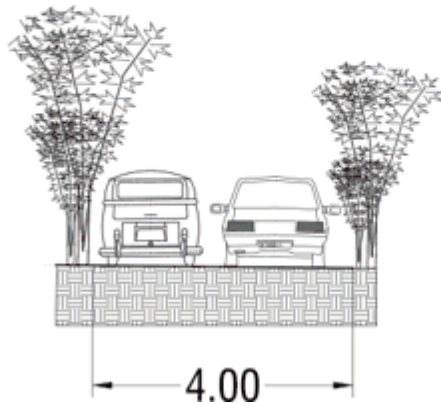
Imagen 40.- Corte del camino de terracería
