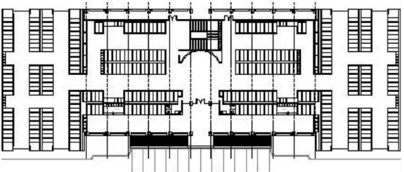
Imagen 16.- Edificio tipo de Mausoleos del Angel
