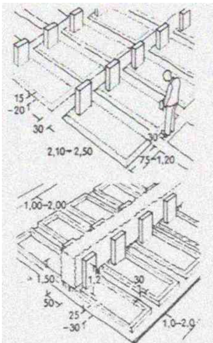
Medidas de áreas del pozo de ataúdes
