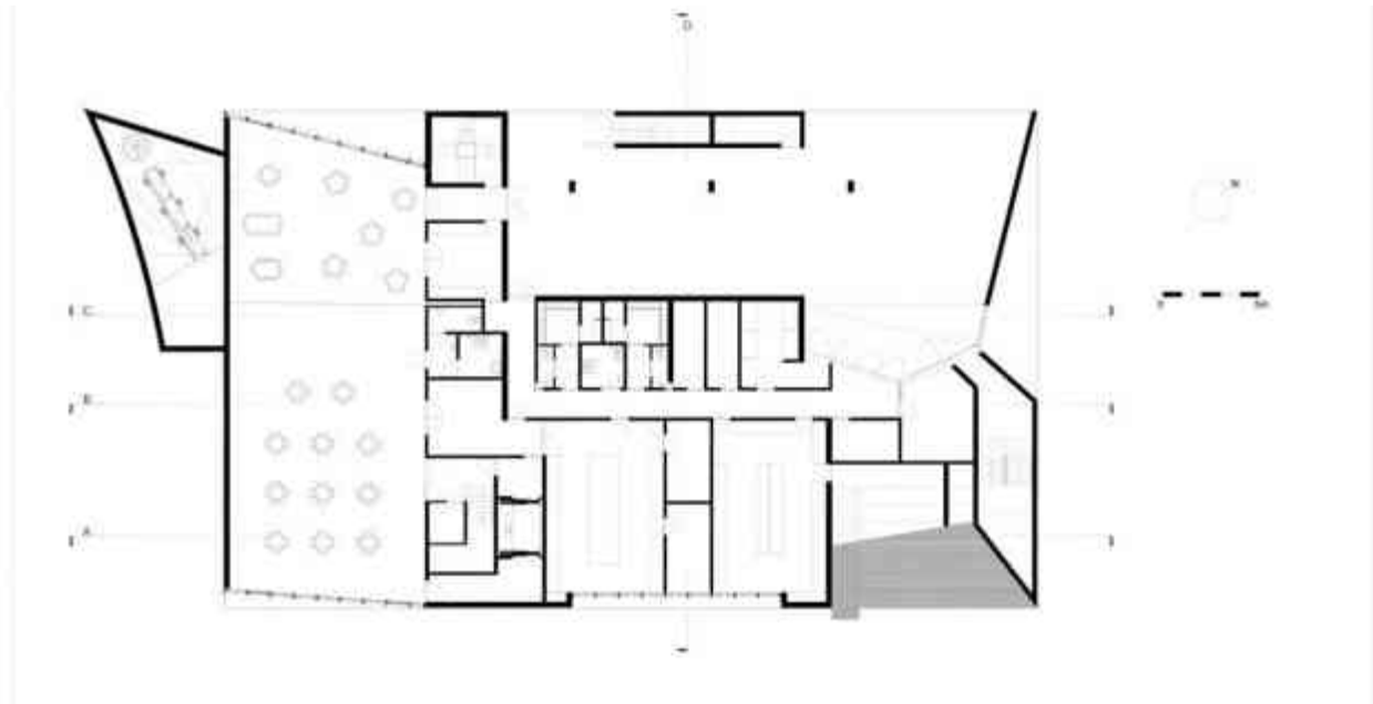
Imágen 46: Planta Primer Nivel Centro Social en Brufe / Imago Recuperado de http://www.archdaily.mx/mx/02-92643/centro-social-brufe-imago 14/10/2014
