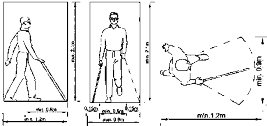
IMAGEN. Medidas antropométricas de persona en silla de ruedas posición estática, (Vista lateral, vista frontal y alzado). 42
