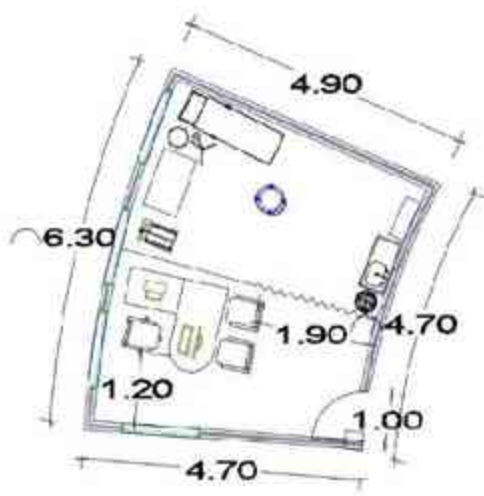
Imagen 91. "Modelo Consultorio" Elaboración: Luna Gómez Surisadday Elizabeth. Abril 2014.
