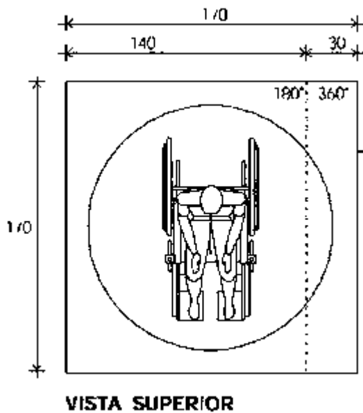
Imagen 83. "Vista superior de silla de ruedas" FUENTE: http://www.libreacceso.org/downloads/discap.pdf f. Consultada: abril 2014
