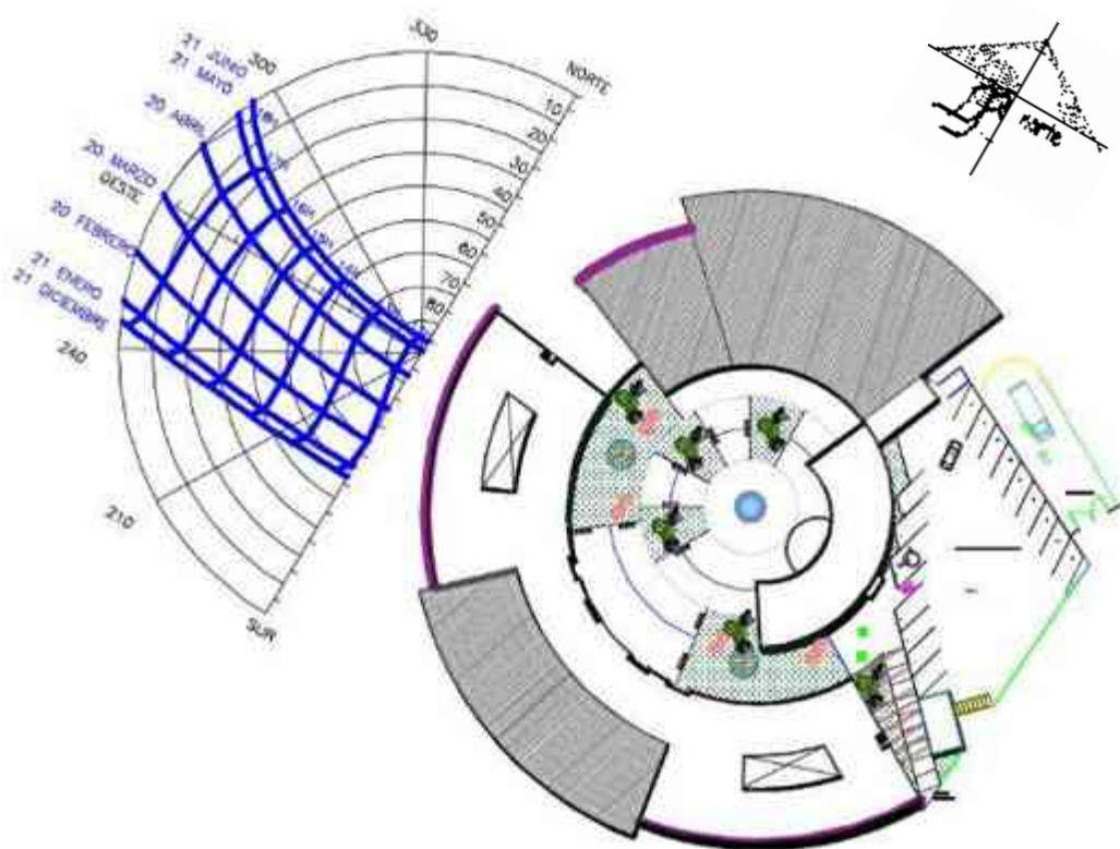
Imagen 68. "Gráfica Solar fachada oeste".Elaboró: Luna Gómez Surisadday E. Elaborado Marzo 2014.
