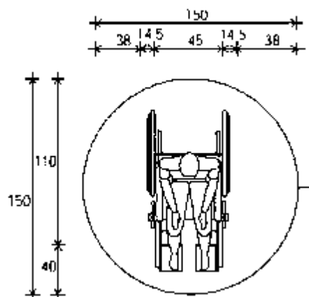
Imagen 84. "Espacio del radio de una silla de ruedas" FUENTE: http://www.libreacceso.org/downloads/discap.pdf f. Consultada: abril 2014
