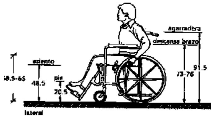
Imagen 82. "Medidas laterales de silla de ruedas" FUENTE: http://www.libreacceso.org/downloads/discap.pdf f. Consultada: abril 2014
