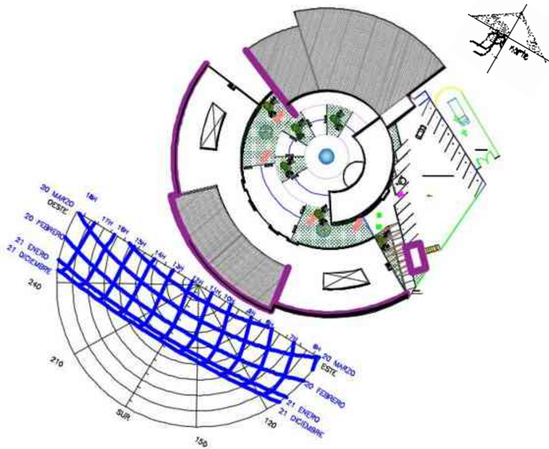
Imagen 66. "Gráfica Solar fachada sur".Elaboró: Luna Gómez Surisadday E. Elaborado Marzo 2014.
