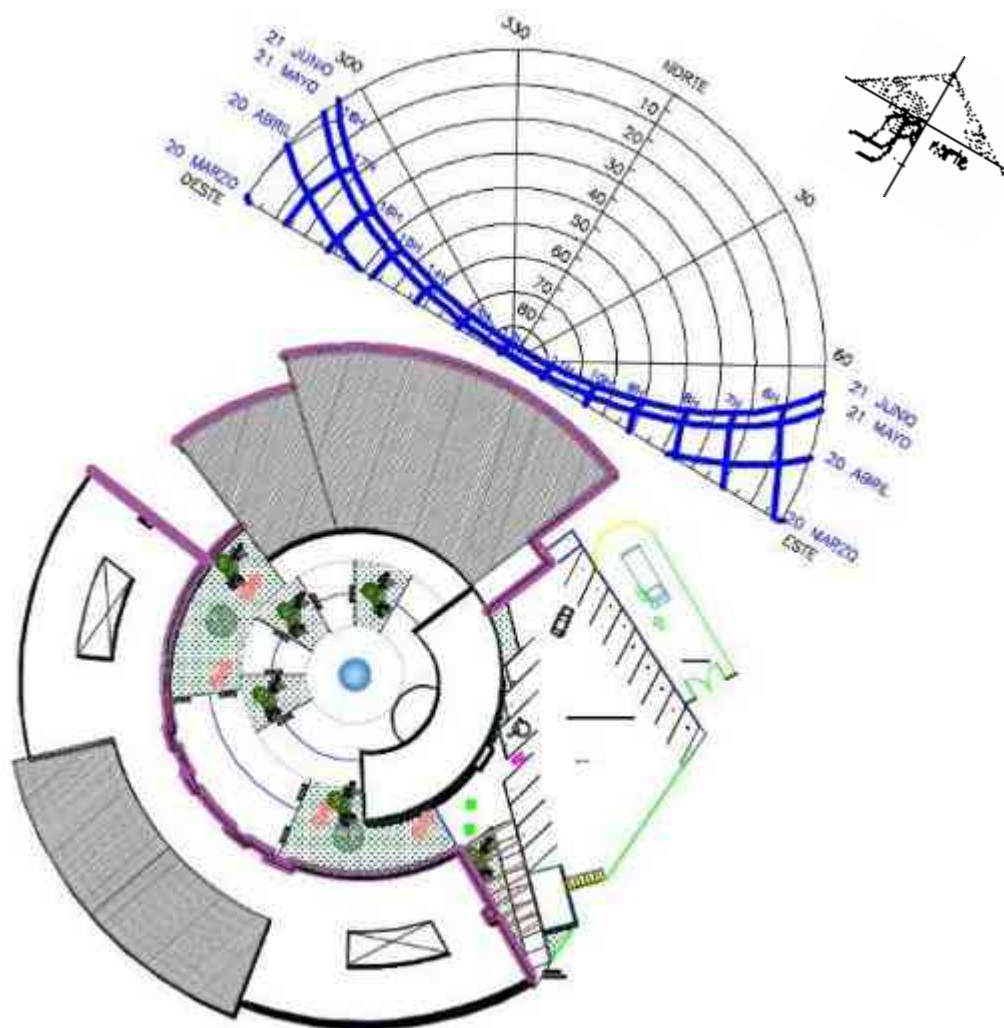
Imagen 65. "Gráfica Solar fachada norte-noreste".Elaboró: Luna Gómez Surisadday E. Elaborado Marzo 2014.
