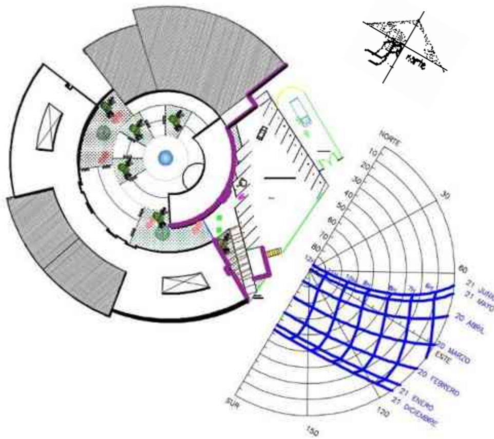
Imagen 67. "Gráfica Solar fachada este". Elaboró: Luna Gómez Surisadday E. Elaborado Marzo 2014.
