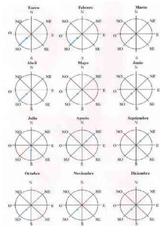
Imagen 63. "Vientos Dominantes".Elaboró: Luna Gómez Surisadday E. FUENTE: http://smn.conagua.gob.mx/index.php?option=com_content&view=article&id=12&Itemid=77 . Fecha de elaboración: Marzo 2014
