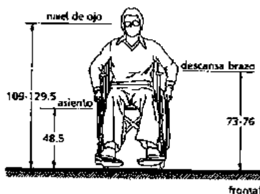
Imagen 81. "Medidas frontales de silla de ruedas" FUENTE:
