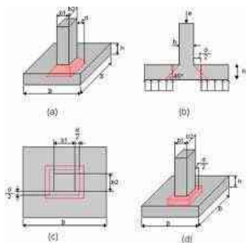
Imagen 77. "Zapatas aisladas". Fuente: http://www.construmatica.com/construpedia/Zapatas_Aisladas . Consultado Marzo 2014.
