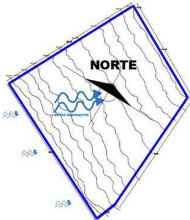
Imagen 64. "Vientos Dominantes en terreno".Elaboró: Luna Gómez Surisadday E. Elaborado Marzo 2014.
