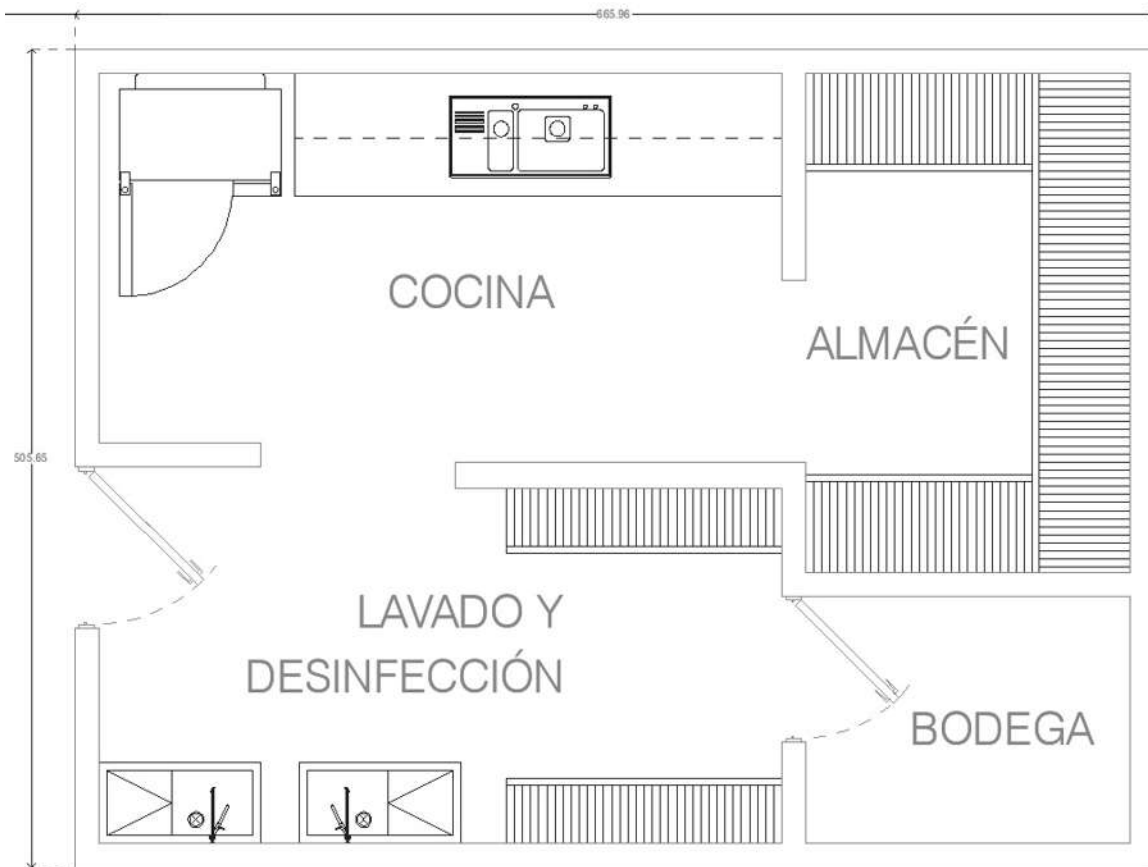
ÁREA DE PREPARACIÓN DE ALIMENTOS SUPERFICIE: 30.25 M 2
