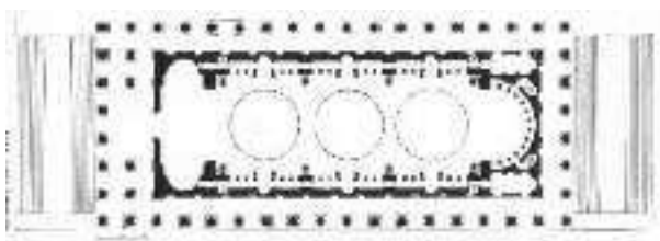
Imagen 17. Planta arquitectónica de la Madeleine de París. Vignon.
