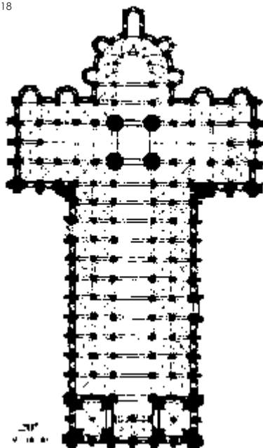
Imagen 9. Planta arquitectónica de La Basílica de Saint-Sernin de Toulouse.
