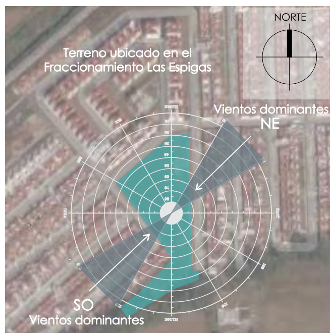
Imagen 32. Relación de vientos dominantes con el terreno.
