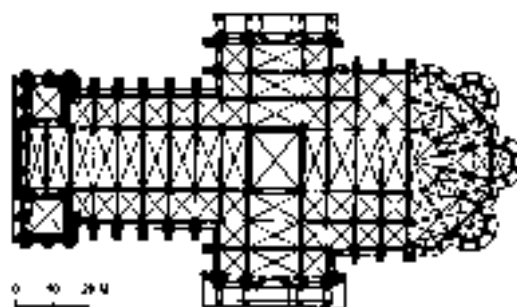
Imagen 11. Planta arquitectónica de la Catedral de Nuestra Señora de París.
