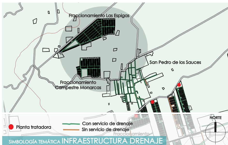
Imagen 40. Infraestructura de drenaje del Fraccionamiento "Las Espigas"
