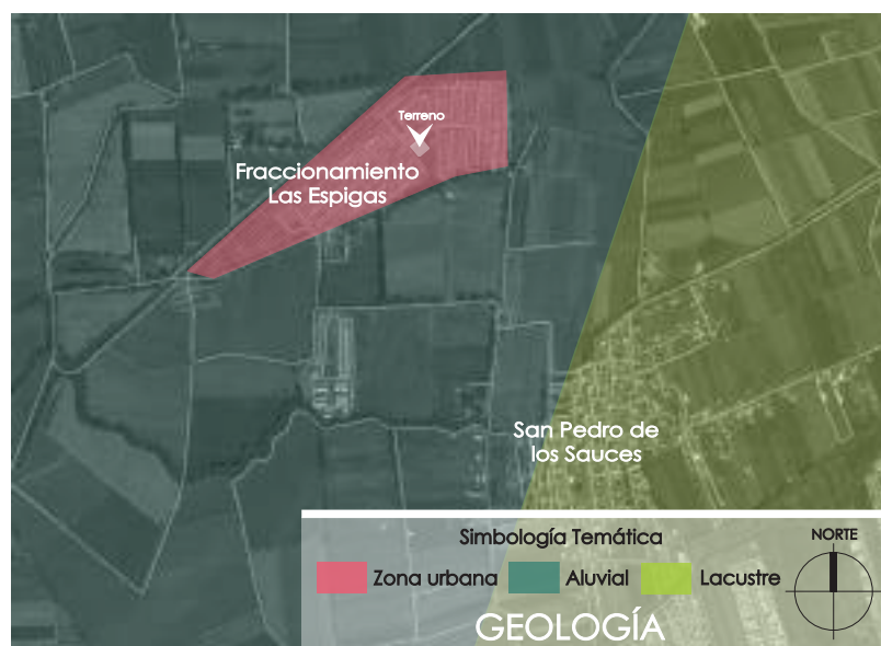
Imagen 26. Geología en el Municipio de Tarímbaro.
