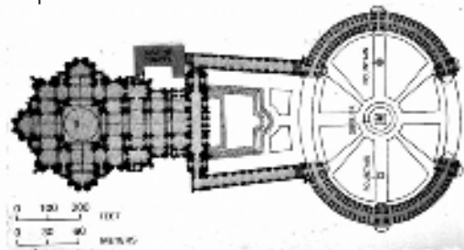
Imagen 15. Planta arquitectónica de la Basílica de San Pedro.
