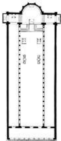
Imagen 7. Planta de la Basílica Santa María la Mayor. Fuente.
