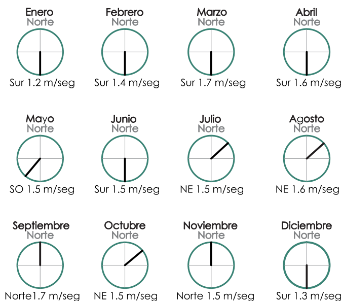
Imagen 31. Vientos dominantes.
