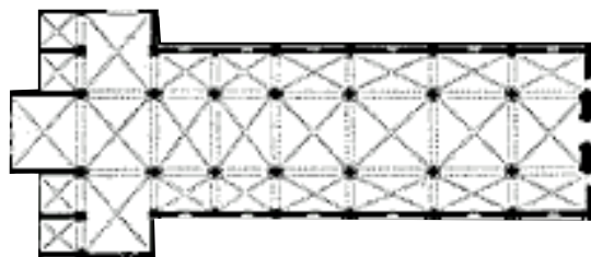
Imagen 13. Planta arquitectónica de la Iglesia de Santa María.
