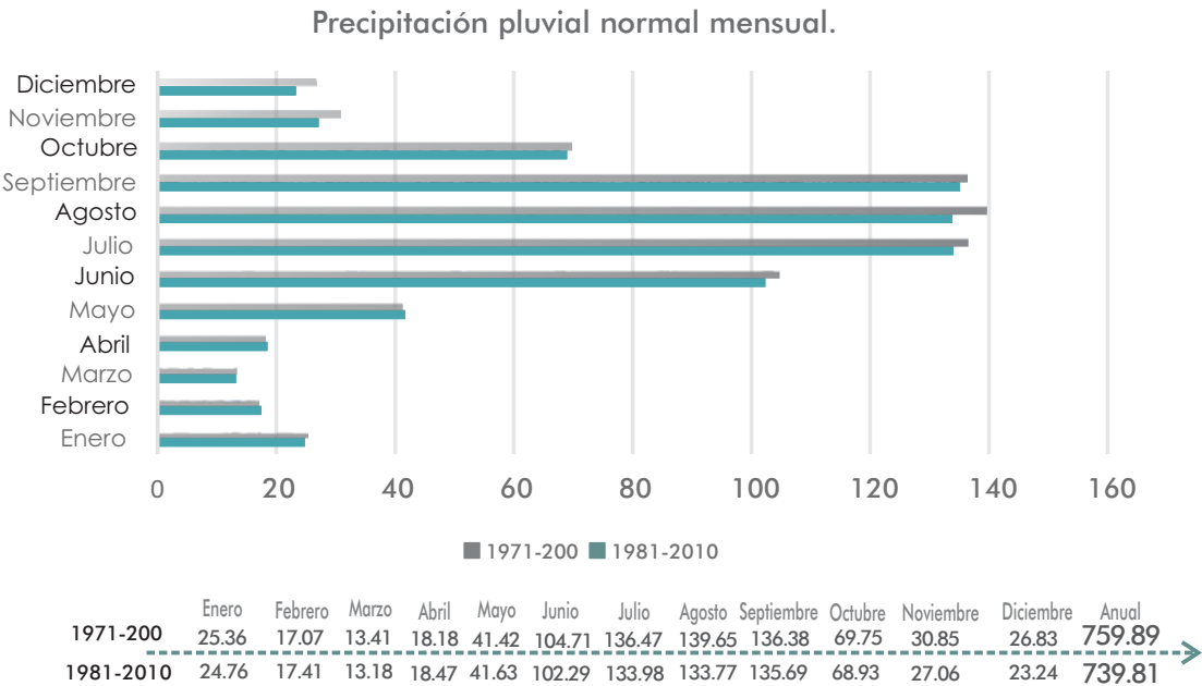
Gráfica 4. Precipitación pluvial en México. Fuente. Elaboración propia con datos del Sistema Nacional de información del Agua
