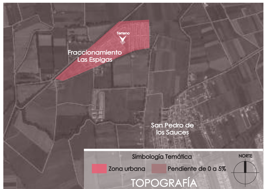
Imagen 30. Pendiente topográfica en el Municipio de Tarímbaro. Fuente. Programa municipal de desarrollo urbano de Tarímbaro.
