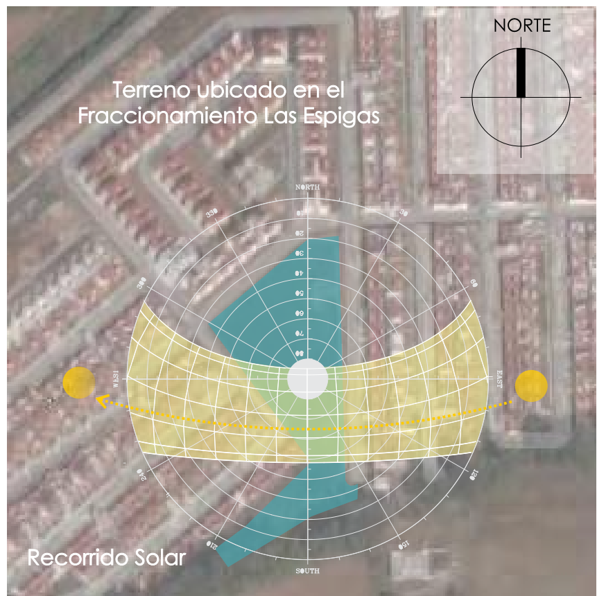
Imagen 33. Gráfica solar del municipio de Tarímbaro. Fuente. Polar sunchart.
