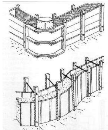
Ilustración U' Ibíd. p. 62. Se muestra algunas variantes de molduras que puede tener el encofrado.
