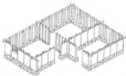
Ilustración C" Ibí., p. 19. Se muestra estructura de bamboo o madera, anclado al sobrecimiento.
