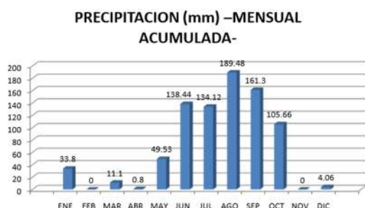
Figure D' Sistema Meteorológico Nacional y Gerencia Estatal de Michoacán de la CNA, 2004.
