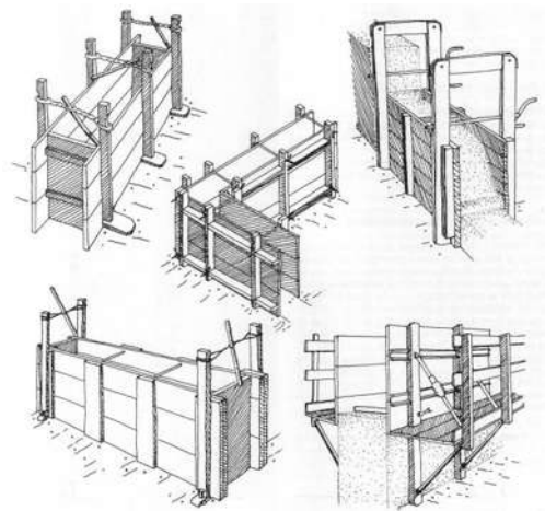
Ilustración T' Imagen tomada de libro de Gernor Minke, p. 60. Se muestra el encofrado.
