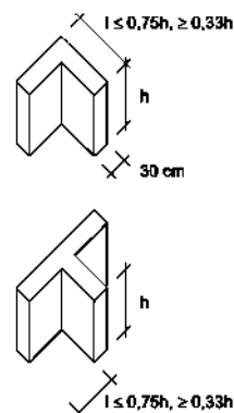
Ilustración Z' Ibíd. p.16. Se muestra la relación de los muros con la altura.
