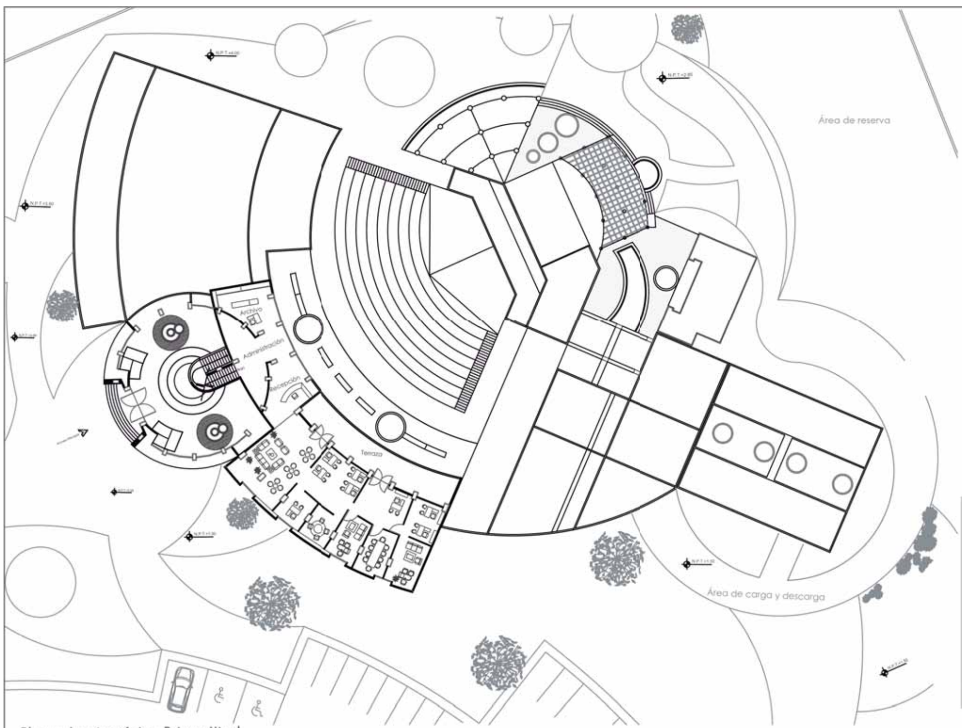
Planta Arquitectónica- Primer Nivel SE
