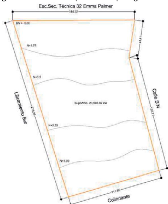
Imagen 6. Croquis del terreno
