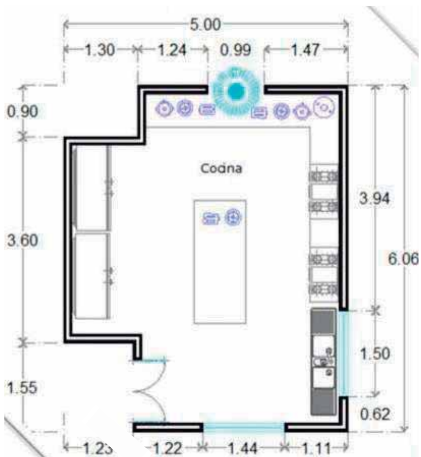
Imagen 15. Cocina, parte del Restaurante
