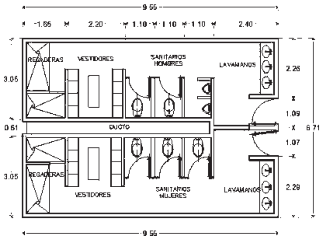
Imagen 16. Dimensionamiento de Sanitarios
