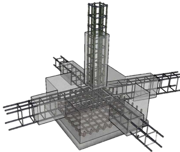
Ilustración 67 zapata aislada central.
