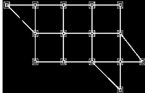
Ilustración 66 zapatas aisladas autor (VBAG)
