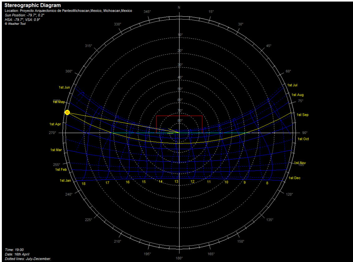
imagen 47. Grafica solar elaborada por Jafet Neftali Cervantes Morales, ECOTEC.
