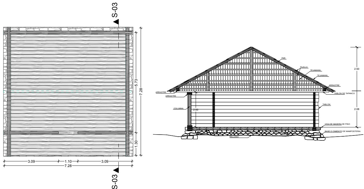
Ilustración 38 Distribución en planta, sección y detalles del troje. Fuente: La troje michoacana, una herencia constructiva, Fecha: Octubre/2018
