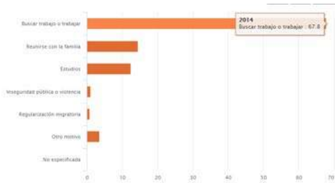
Gráfica 2 Distribución porcentual de emigrantes internacionales por causa de la emigración,
