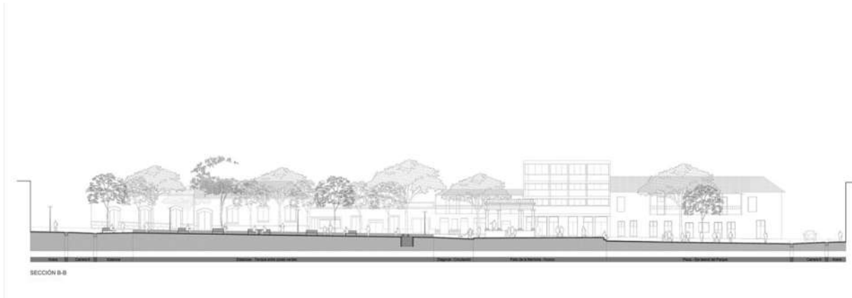
Ilustración 25. Recuperación del parque principal Agueda Gallardo/Arquitectura y espacio urbano, corte 2, recuperado de https://www.archdaily.mx/mx/792706/recuperacion-del-parque-principal-agueda-gallardo-arquitectura-y-espacio-urbano/57a32762e58ece1e3d0000f6-recupera
