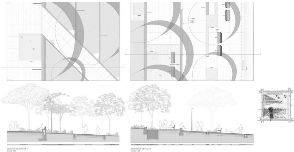
Ilustración 27. Recuperación del parque principal Agueda Gallardo/Arquitectura y espacio urbano, detalle 2, recuperado de https://www.archdaily.mx/mx/792706/recuperacion-del-parque-principal-agueda-gallardo-arquitectura-y-espacio-urbano/57a3277ce58eced3c70000e2-recuper
