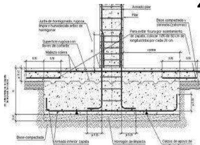
Fig.30. Zapatas aisladas – representación de construcción https://sites.google.com/site/representacionconstruccion/06-unidad-6/05-zapatas-aisladas . F de Rec 09/2019.
