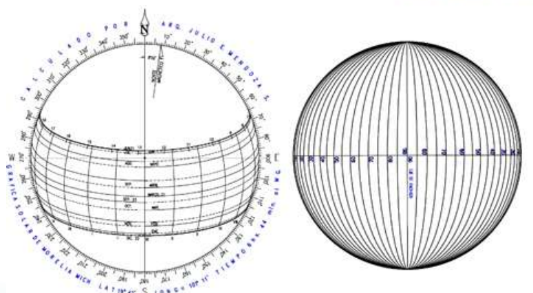
Ilustración 7 trayecto del sol, obtenido: FUENTE: https://dokumen.tips/documents/grafica-solar-morelia-mich-model.html consultado: 5 noviembre 2020
