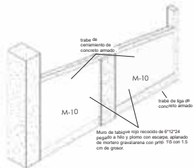
4 Detalle de M-10.
