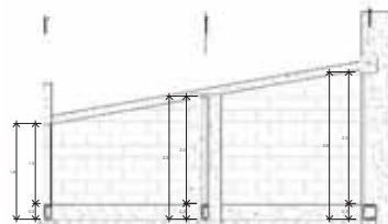
5 Corte trasversal. 1 : 50
