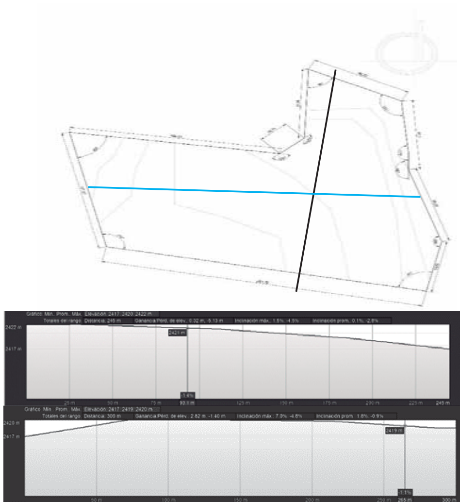
Corte longitudinal.
