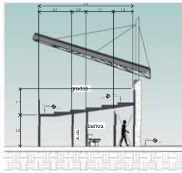
① corte transversal area de gradas. 1:75
