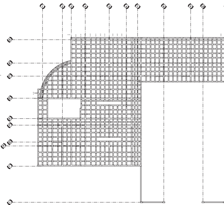
4 Losa nervada area administrativa. 1 : 100
