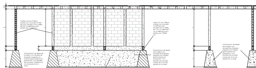
58 corte Y-Y' 1 : 50
