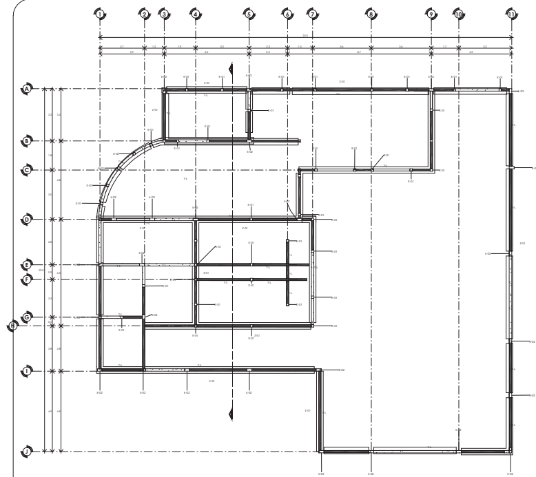
1 Estructura area administrativa. 1 : 100
