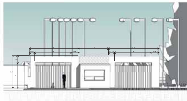
② Fachada de acceso vehicular. 1:75
