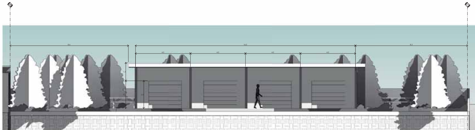
④ corte transversal area de vanas-comedores. 1:50
