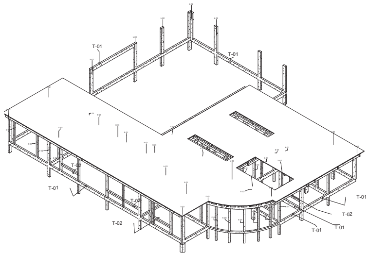
2 isometrico de estructura 1.
