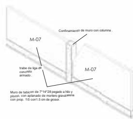
3 Detalle de union M-07
