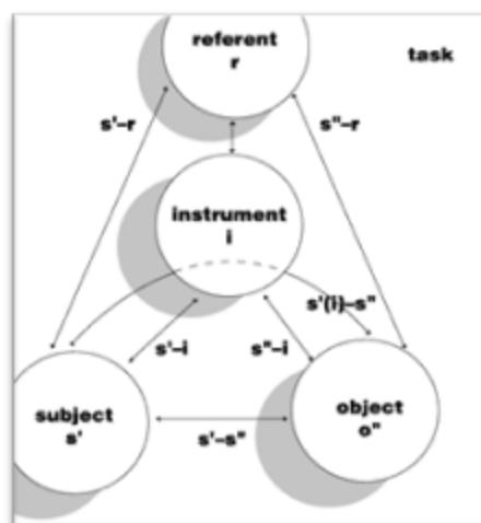
Figura 3: Modelo SIA modificado
