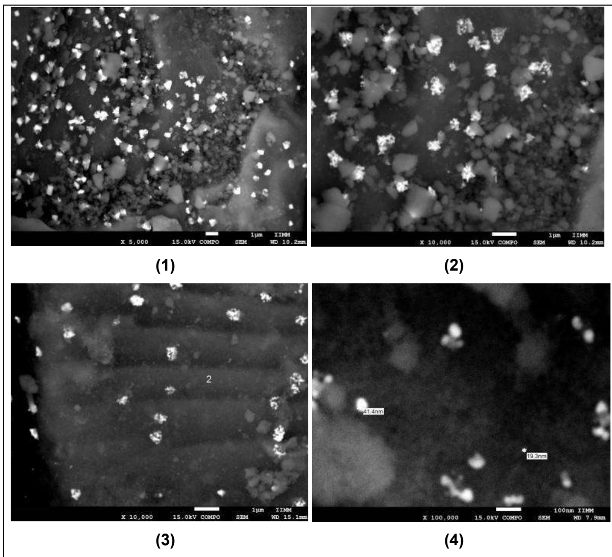
FIGURA 14 Micrografías de Ag/TiO 2 con energía UV (1)5000X, (2)10000X, (3)10000X Y (4)100000X.
