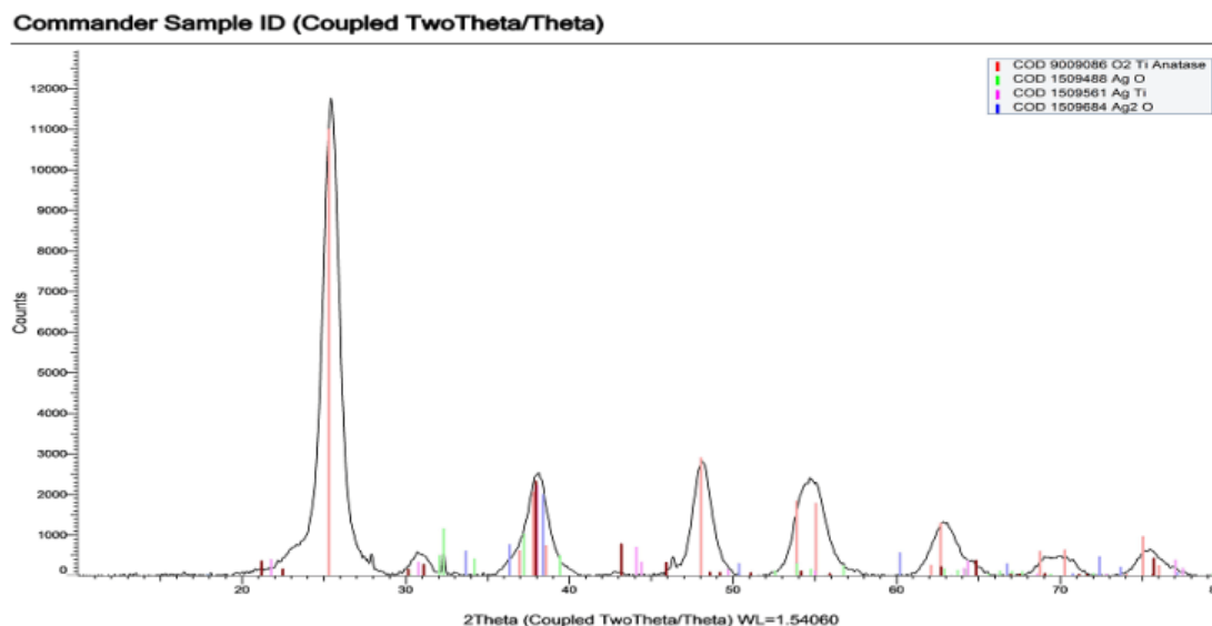
FIGURA 16 Difractograma DRX de la muestra \text{TiO}_2\text{-Ag}
