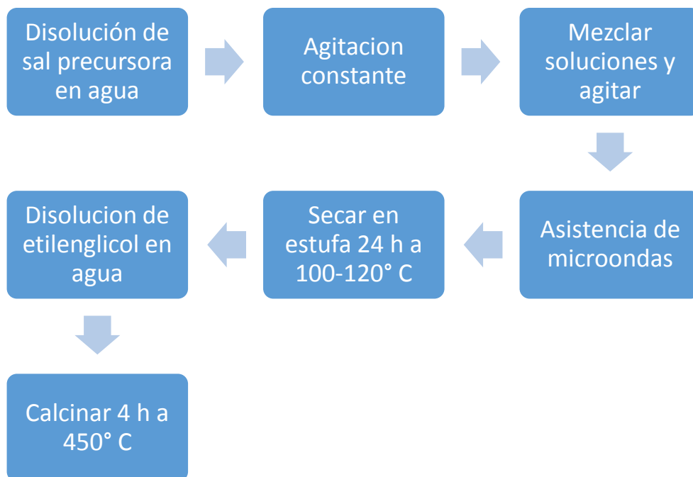
Figura 6 Diagrama general de síntesis sol-gel de \text{TiO}_2 .
