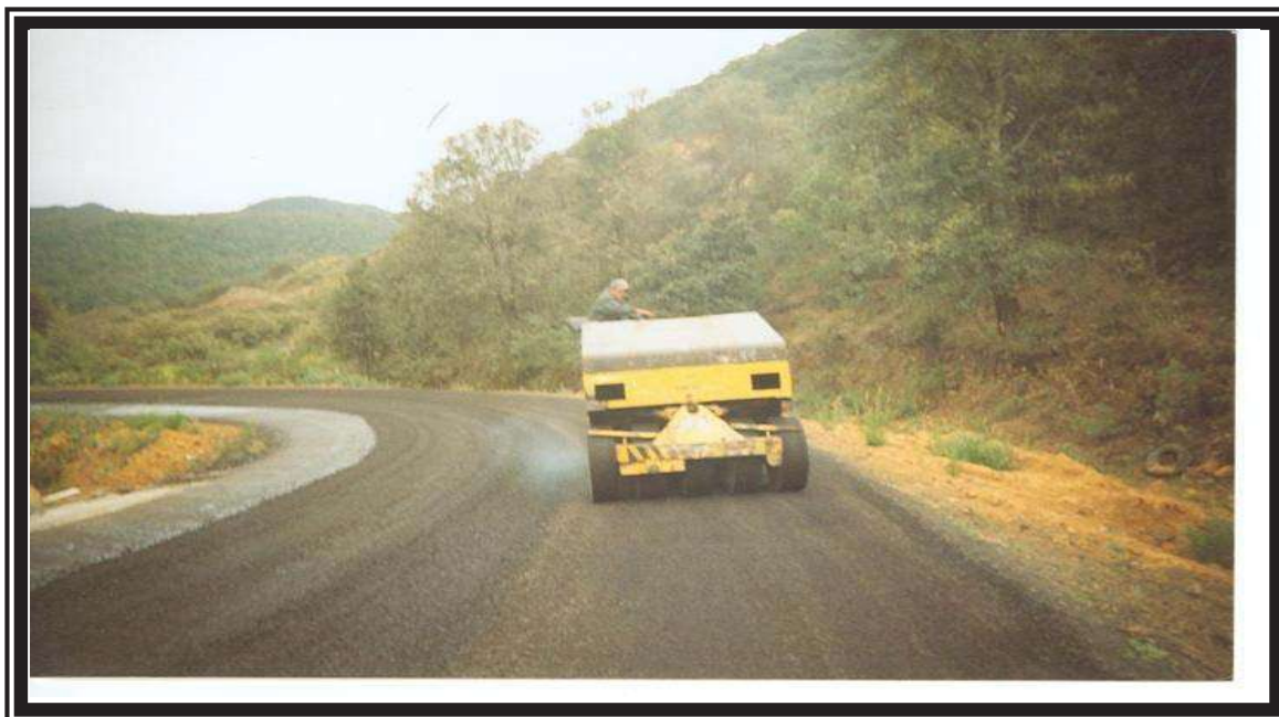
FOTO No.27 APLICACIÓN DEL RIEGO DE SELLO.
