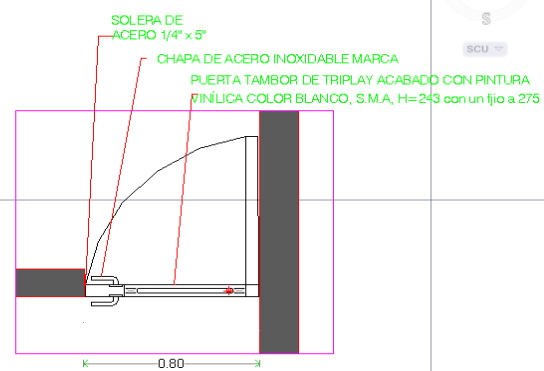
P2- PUERTA TIPO 2
