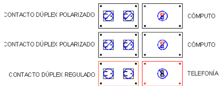
DETALLE DE NÚCLEO TIPO C PLANTA
