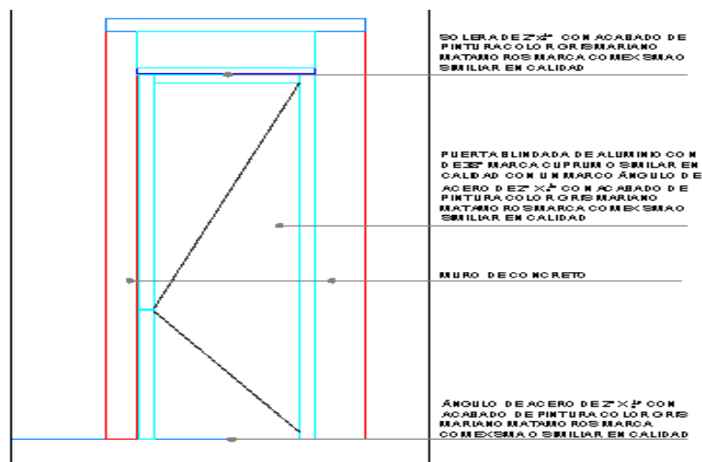
CAN-06 ALZADO
