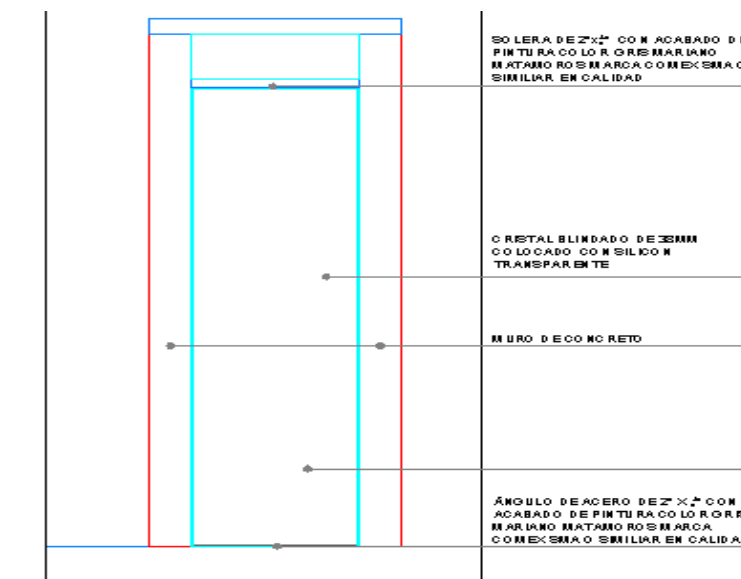
CAN-05 ALZADO
