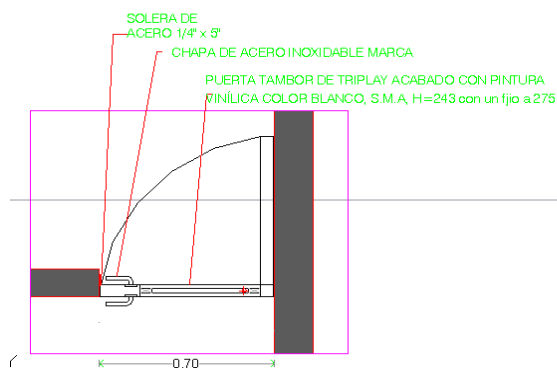
P1- PUERTA TIPO 1
