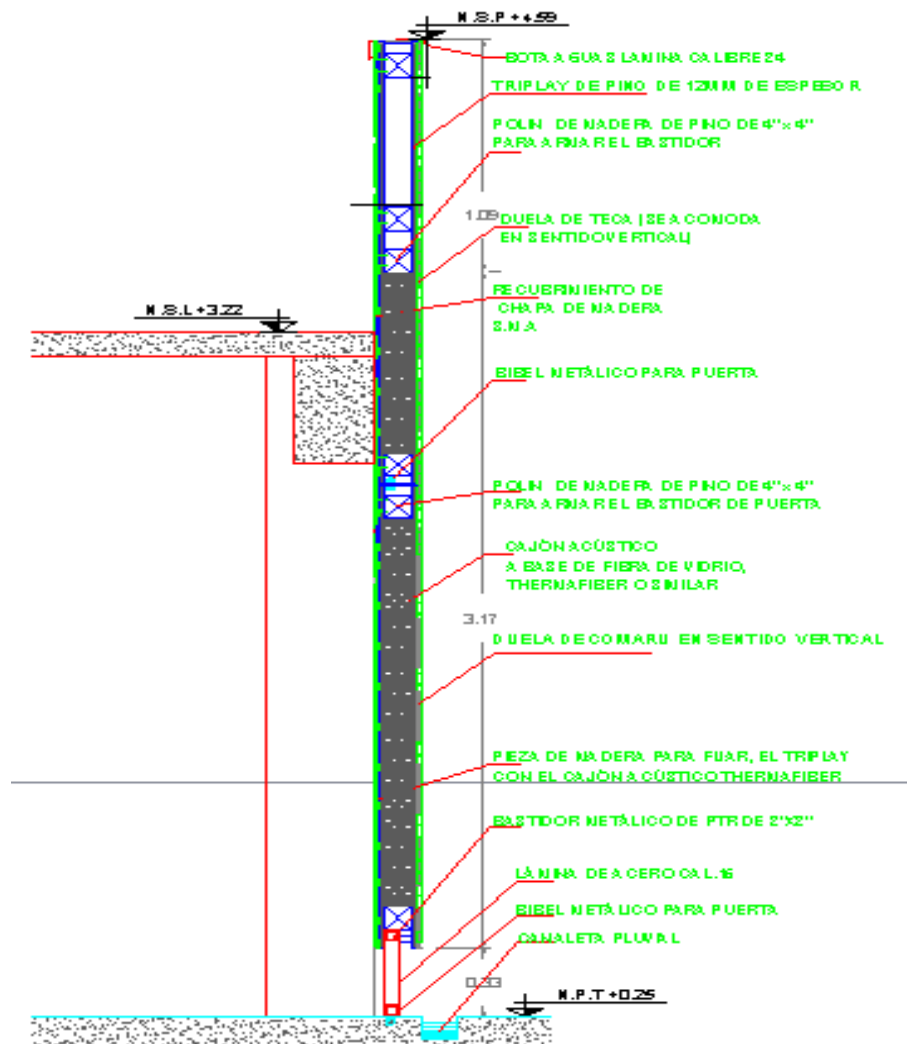
DETALLE DE MURO DE SALA DE AUDIENCIA P3- PUERTA TIPO 3
