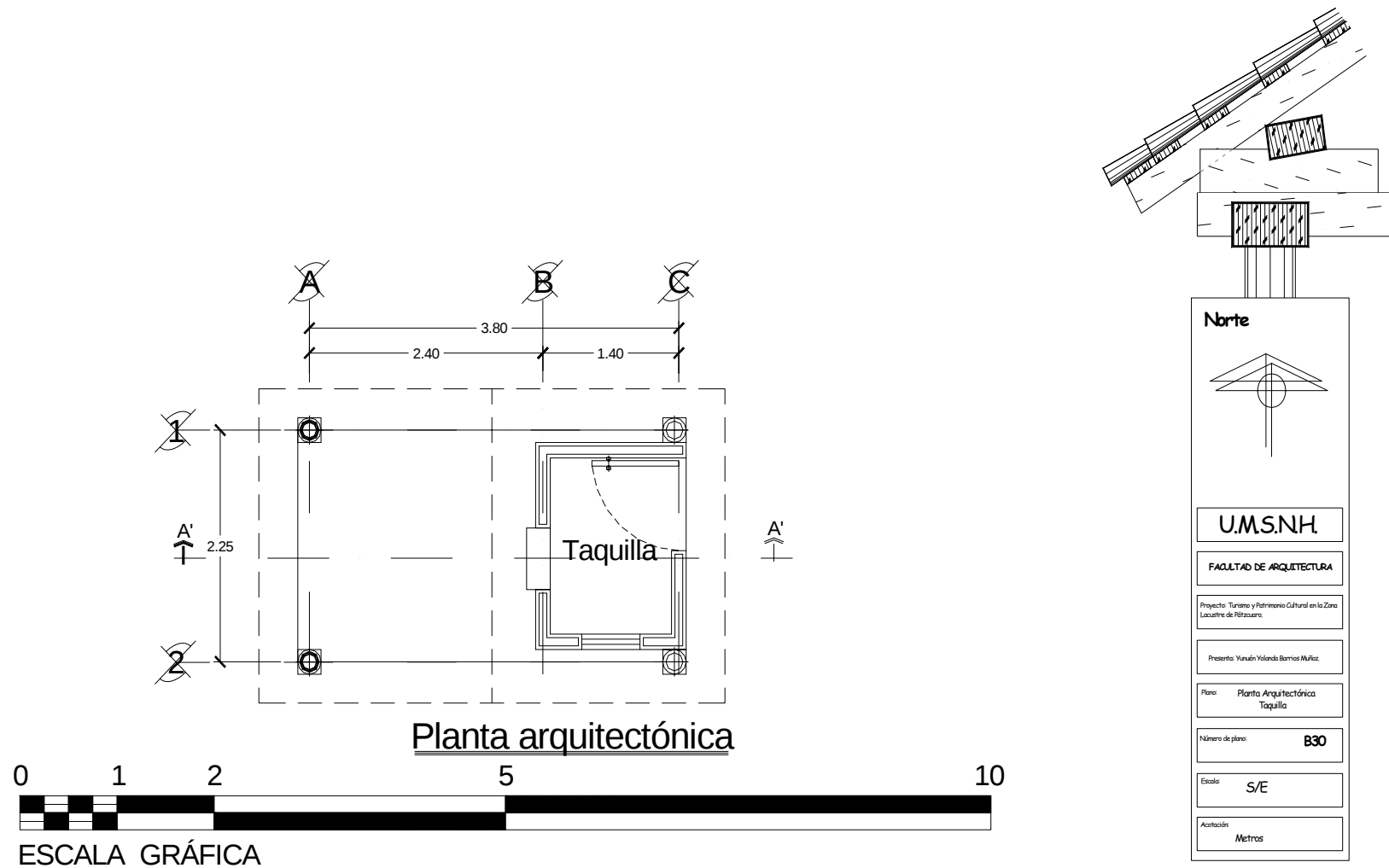
PLANTA DE AZOTEAS TAQUILLA.
