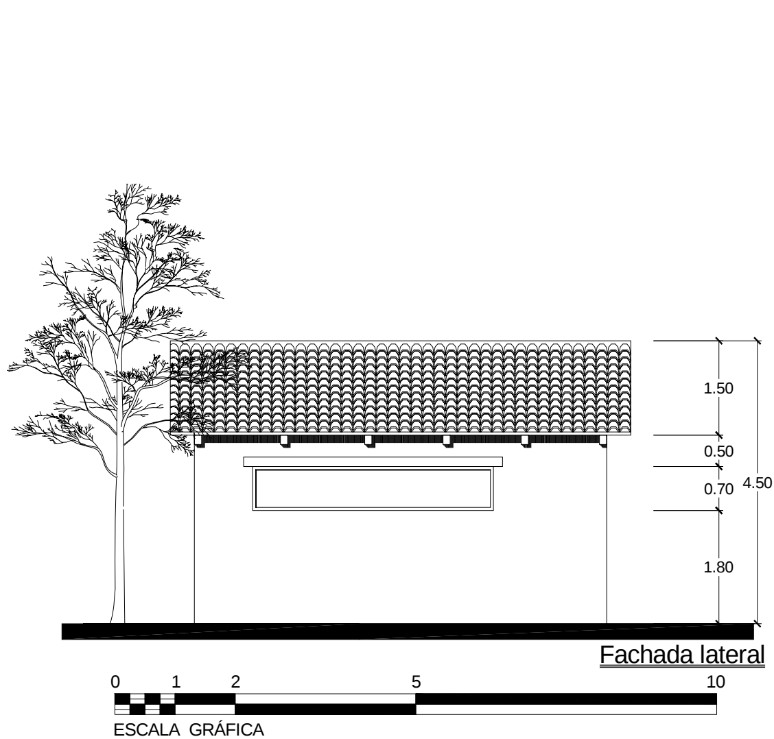
CORTE A-A' SANITARIOS TIPO.
