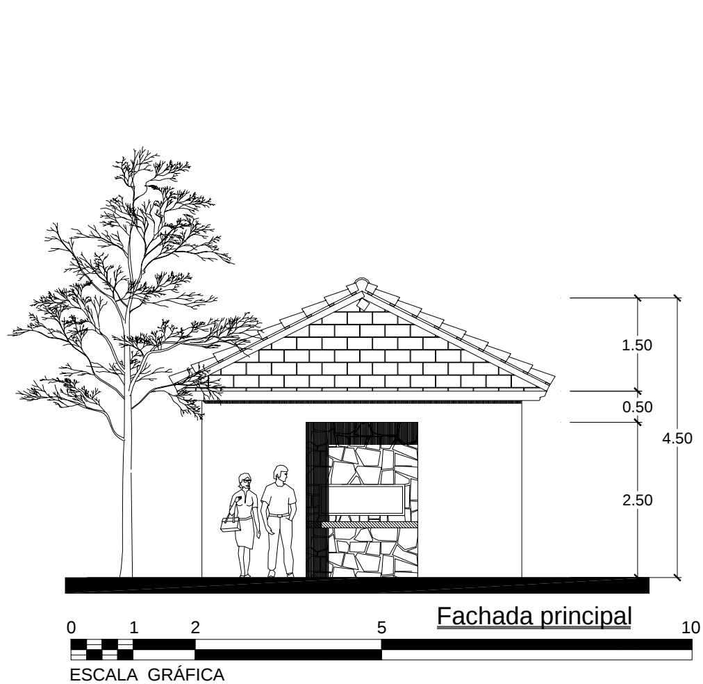
FACHADA LATERAL SANITARIOS TIPO.
