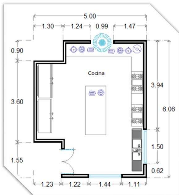
Imagen 68. Prototipo de cocina para el servicio de 150 personas. Con espacio para estufa, fregadero, refrigeración y mesa de maniobras. En una área de 27 m 2 .
