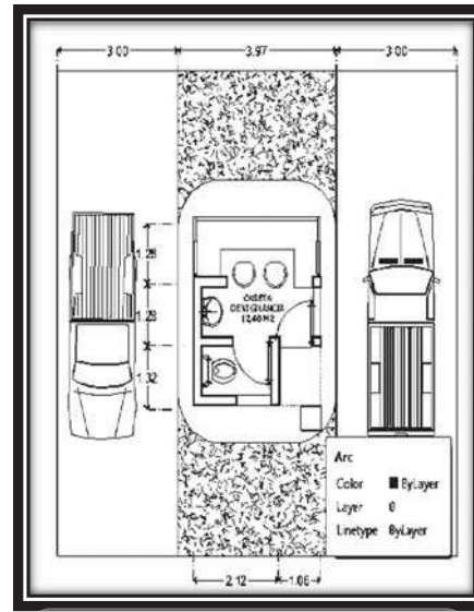
Imagen 70. Análisis del área de acceso a través de una caseta de vigilancia en dos sentidos. Resuelto en 20 m2.
