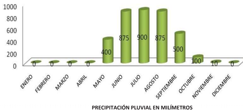
Imagen 51. Precipitación pluvial mensual, considerados los meses de mayo, junio, julio y agosto, con la mayor precipitación; en cuanto al diseño del proyecto no fue un obstáculo para el empleo de terrazas y losas planas.
