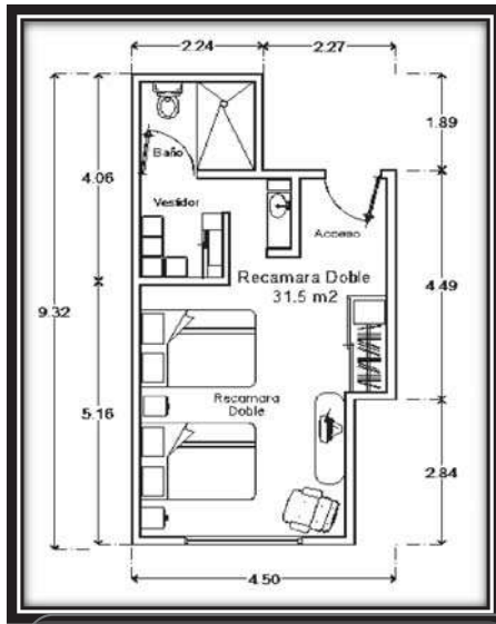
Imagen 69. Espacio requerido para el diseño de las cabañas representando una recámara para cuatro personas, con closet y baño- vestidor, en 21.50 m2 construidos
