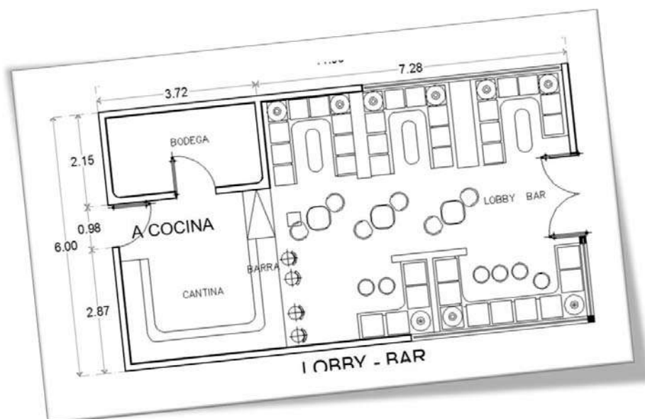
Imagen 67. Señala la cocina requerida para lobby-bar y fuente de soda con barra de servicio a clientes en un área de 66 m 2 .
