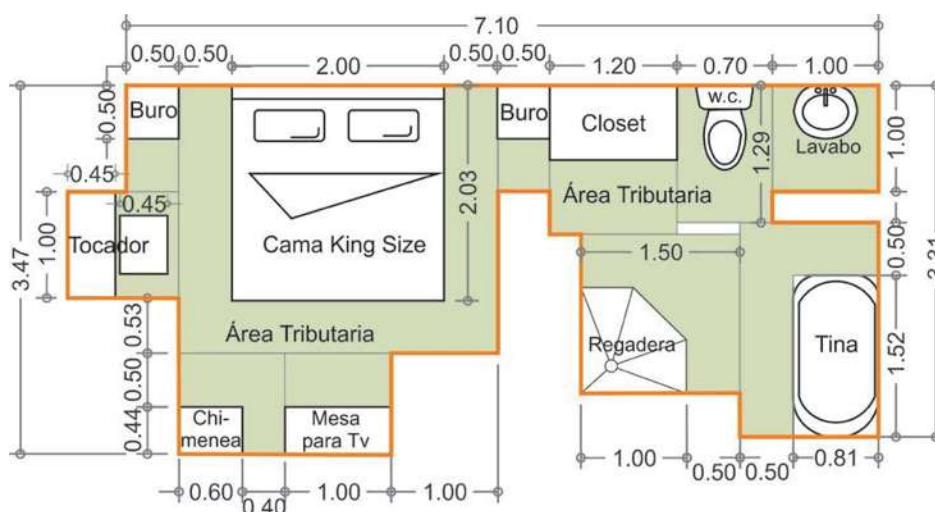
Croquis número 14, cotas en metros y sin escala
