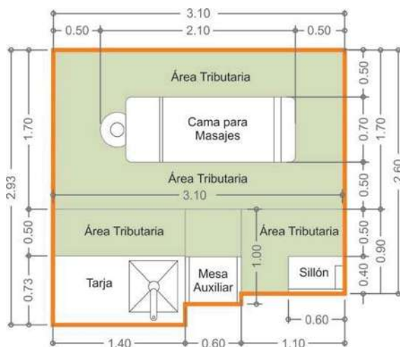
Croquis número 10, cotas en metros, sin escala.
