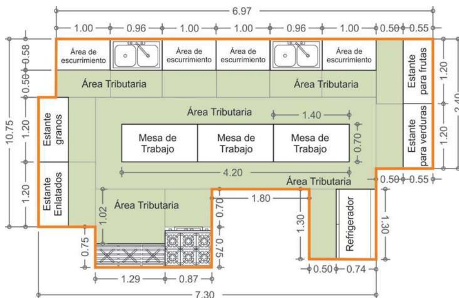
Croquis número 13, cotas en metros y sin escala.
