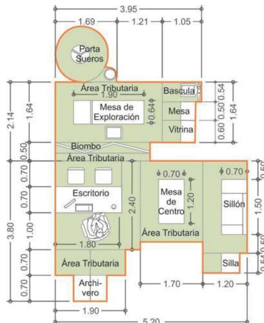
Croquis 12, sin escala y cotas en metros
