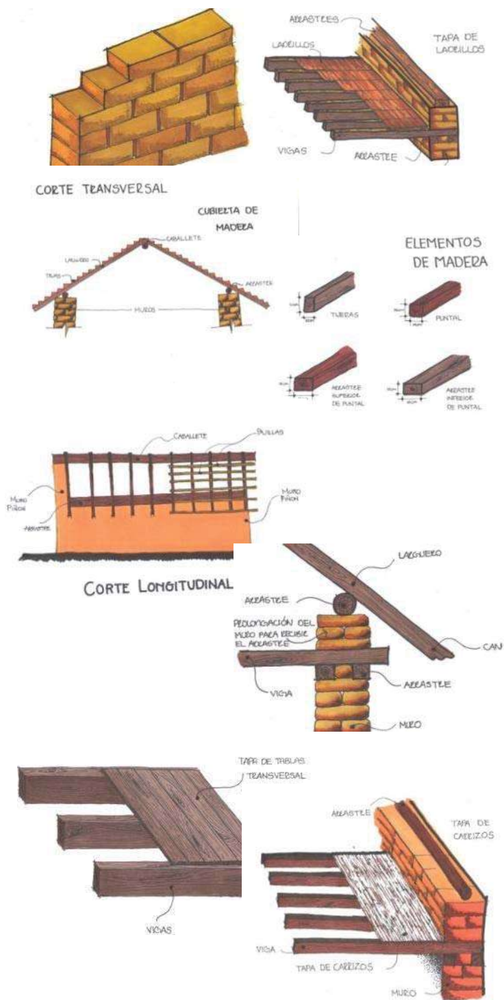
200/detalles de procedimientos y materiales constructivos/ SUMA, Departamento de Conservación e Imagen Urbana/2011
