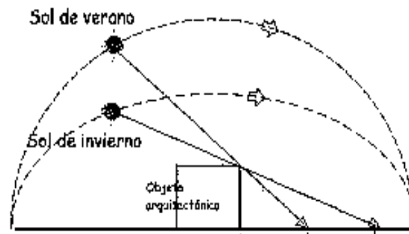
Imagen 3.3 Diferencia de proyecciones de sombra en verano e invierno. Imagen obtenida en [http: //franciscobrun.googlepages.com/asoliamento.jpg/asoliamentofull.jpg,
