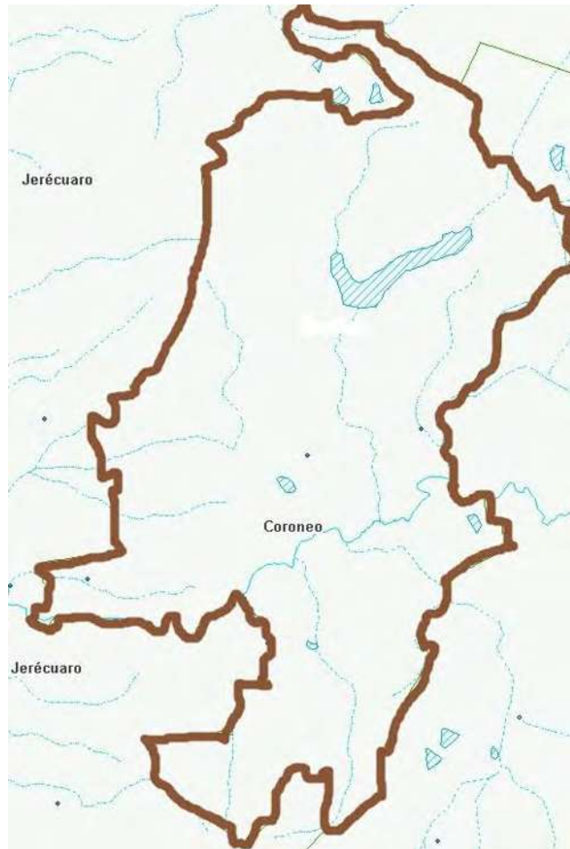
Imagen 3.4 HIDROLOGIA DEL MUNICIPIO DE CORONEO Imagen Obtenida De INEGI. Mapa Digita 5. Proyecto Información Básica. Modificada Por Imelda Gpe. Pérez
