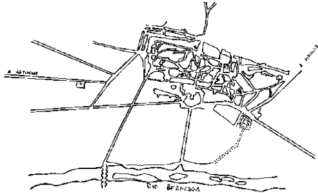
Imagen 1.7 León, España en el Siglo XIX, ubicación del Cementerio de León en las afueras de la ciudad, al norte del núcleo habitado, dando seguridad de que los vientos dominantes del noreste no llevarían a la ciudad aires viciados.
