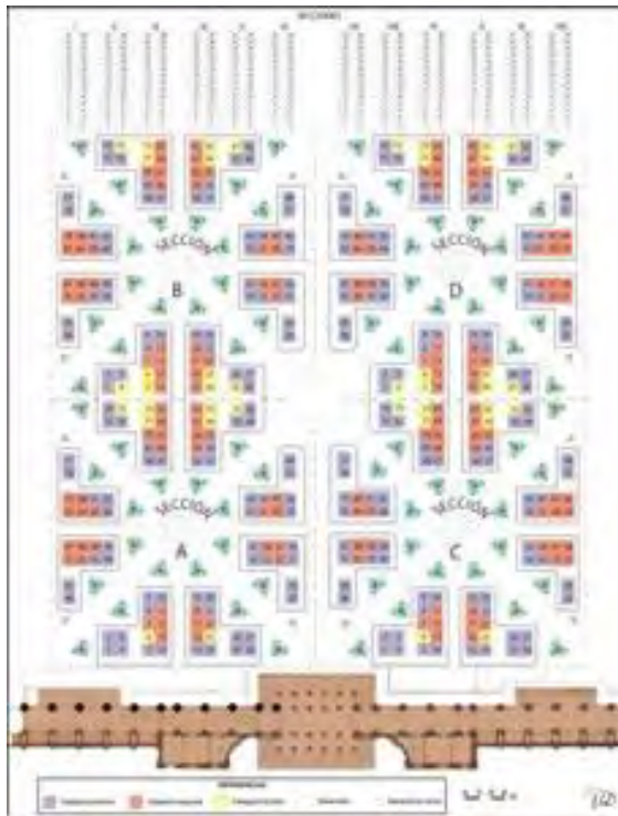
Imagen 1.24 Plano arquitectónico del cementerio de La Plata. Imagen obtenida de http://www.municipalidad.laplata.gov.ar/areas/secretariagestionpublica/173-cementerio-de-la-plata
