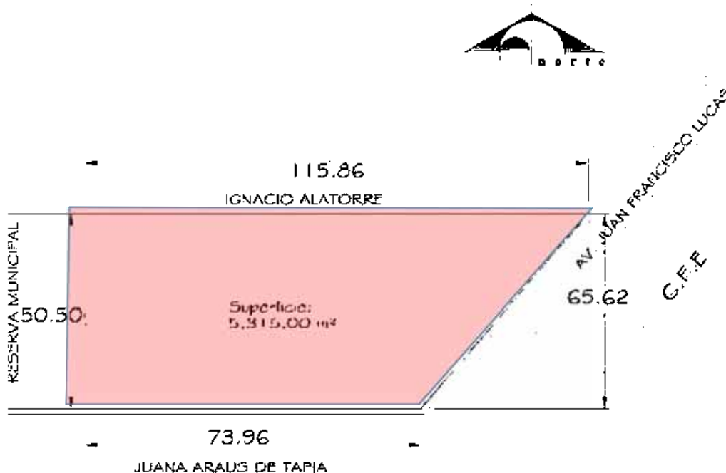
Imagen 14. Croquis con el área del terreno, sus colindancias y dimensiones. Por Patrimonio del Municipio
