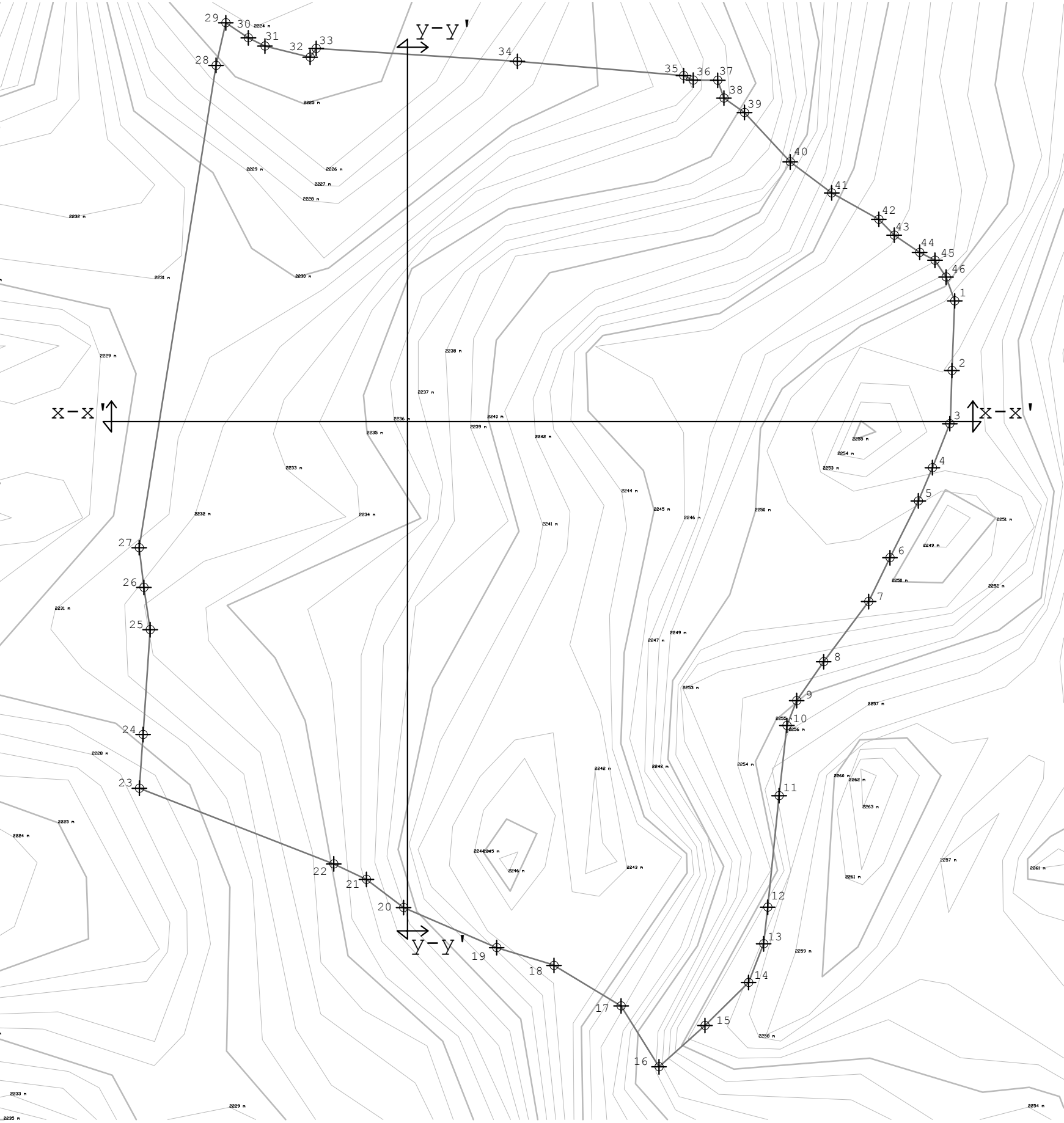
POLIGONAL CON CURVAS DE NIVEL
