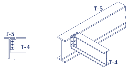
DETALLE DE ARMADO DE LOSACERO.
