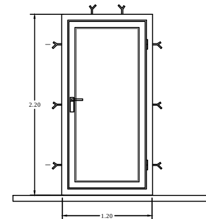
P.P.S.-01 PUERTA -02 de cancelería de aluminio, color café madera.
