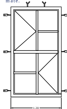
V.T.LLR-01 VENTANA TALLER de herrería, color negro mate.
