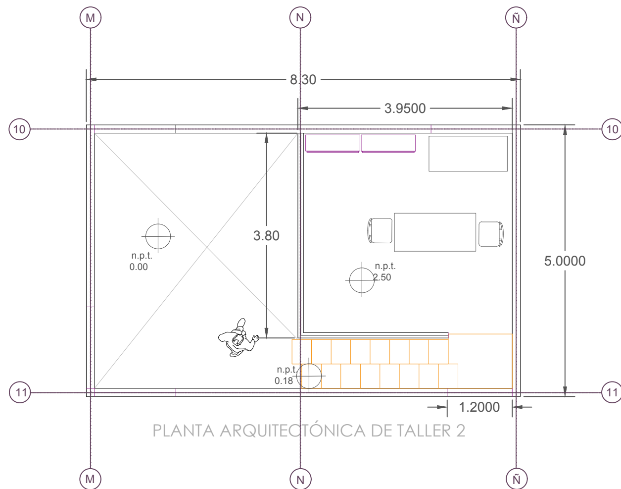
PLANTA ARQUITECTÓNICA DE TALLER 2
