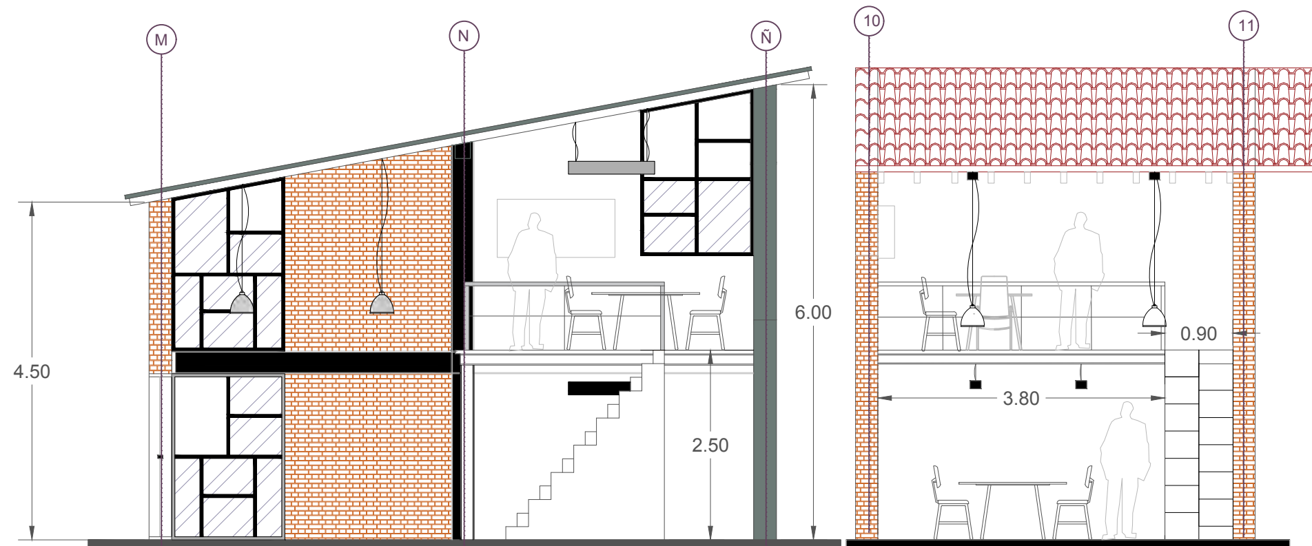
CORTE a-b DE TALLER 2
