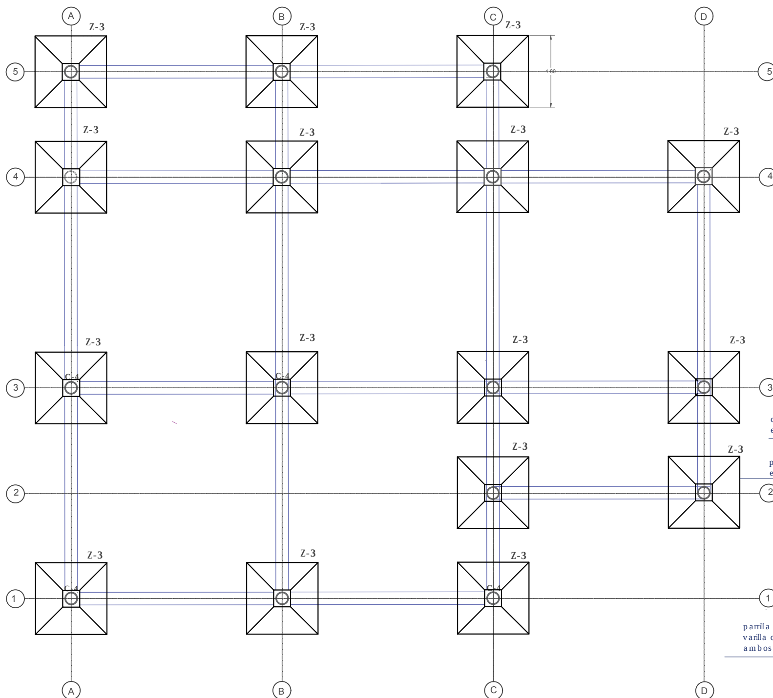
CIMENTACIÓN DE GALERÍA.
