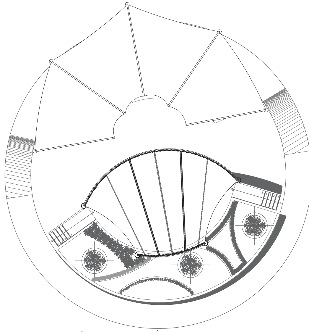
PLANTA ARQUITECTÓNICA DE TEATRO AL AIRE LIBRE, CON TECHO DE LONA.
