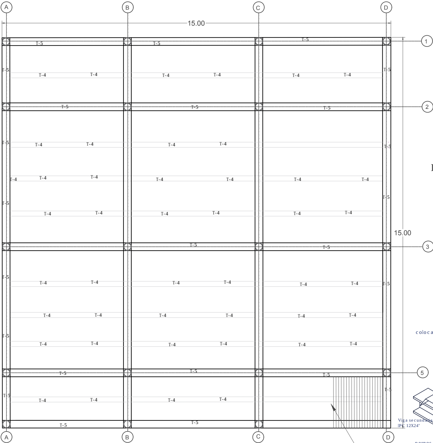
DETALLE DE LOSACERO
