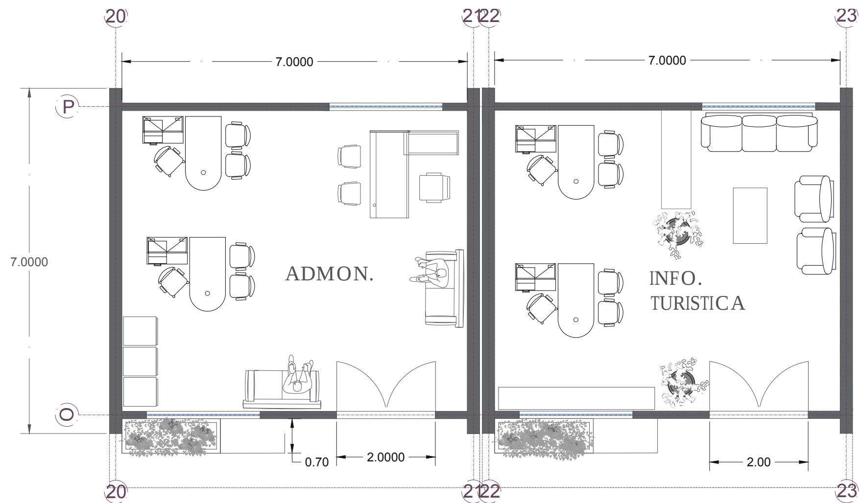
PLANTA ARQUITECTONICA DE ADMINISTRACION E INFORMACION TURISTICA.
