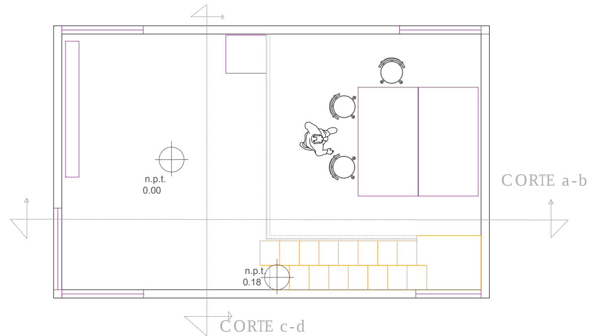
PLANTA ARQUITECTÓNICA DE TALLER 2
