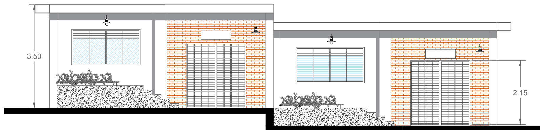
FACHADA DE ADMON. E INFO. TURISTICA
