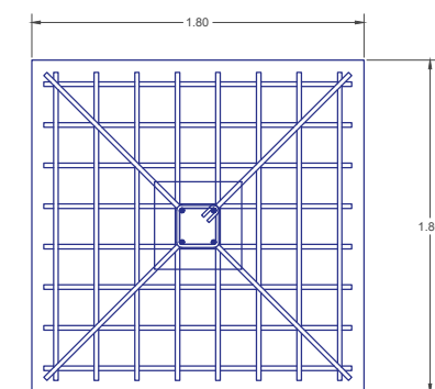
DETALLE DE ARMADO DE ZAPATAS.
