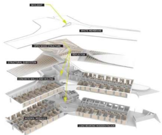
Fig. 63. Albergue juvenil en Bayreuth, Alemania. Consulta: 17/09/17. Fuente: LAVA. 2014
