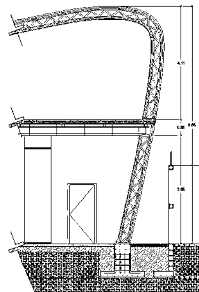
CF-01 Corte por fachada 1
