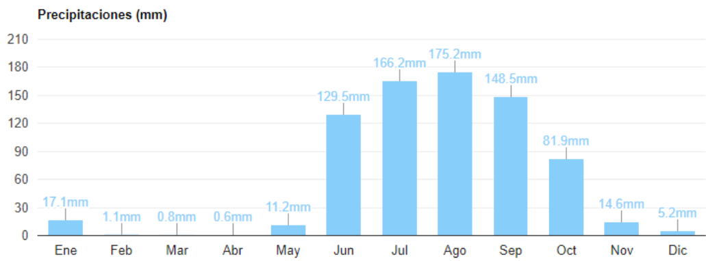
Fig. 23. Gráfica de precipitación pluvial anual. Consulta: 23/10/17. Fuente: Weather Atlas.
