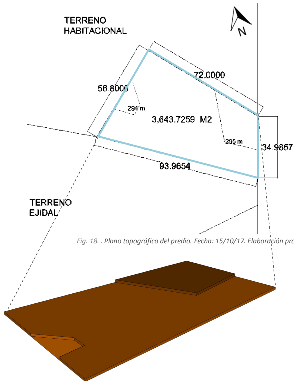
Fig. 19. Topografía del terreno en vista 3D. Fecha: 15/10/17.
