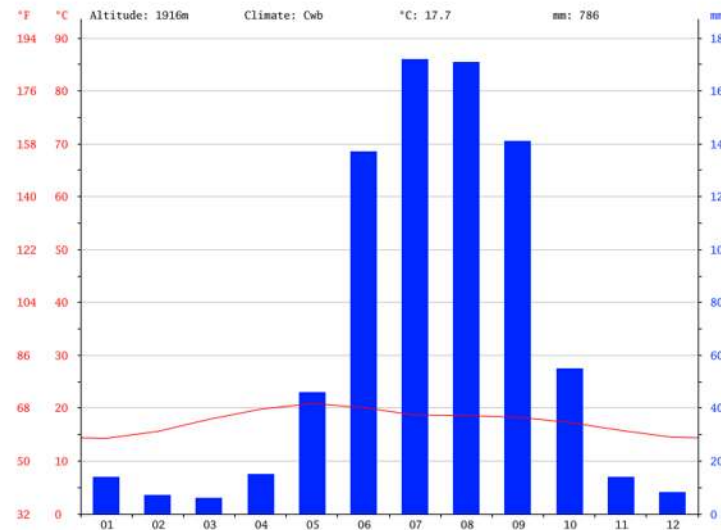
33 | Gráfica de precipitación pluvial en Morelia
