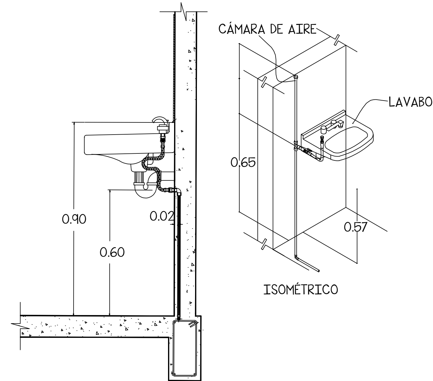
DETALLE DE ALIMENTACIÓN DE LAVABO
