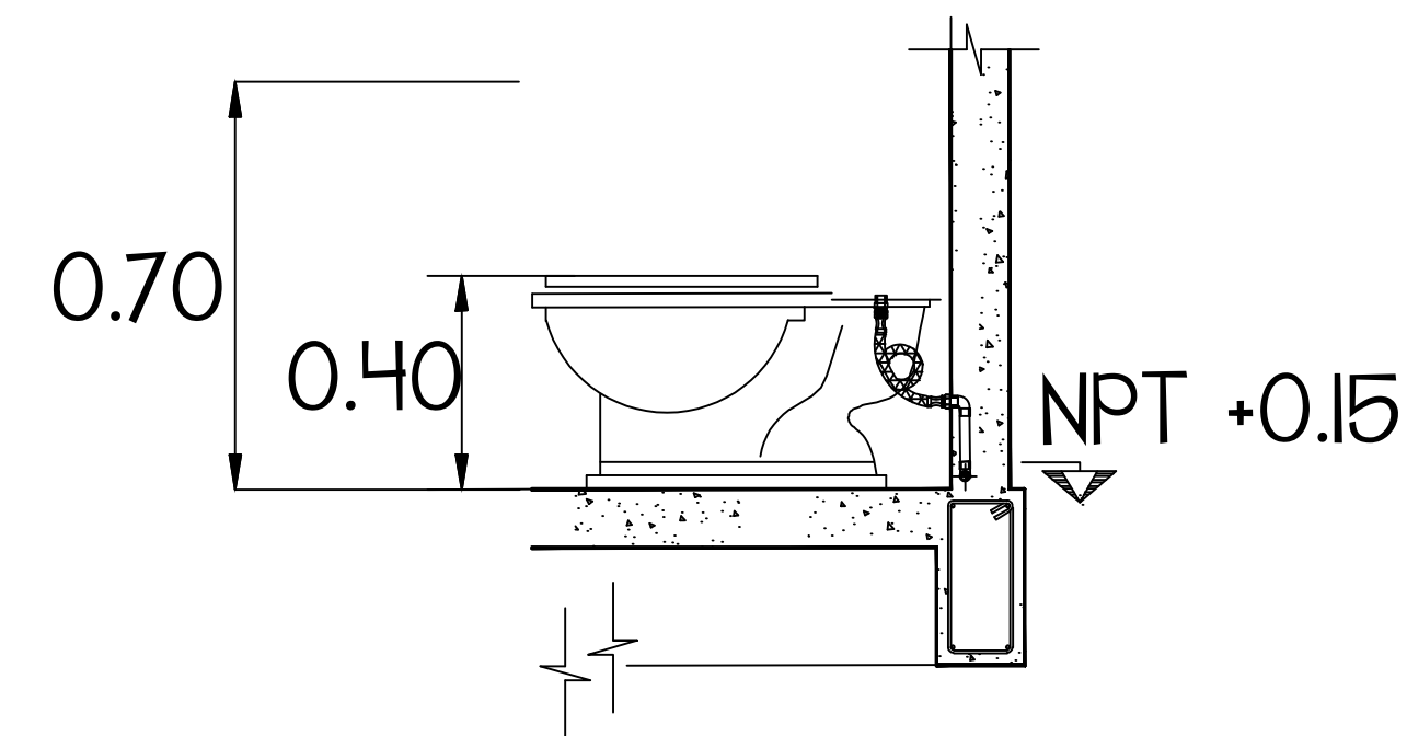
DETALLE ALIMENTACIÓN W.C
