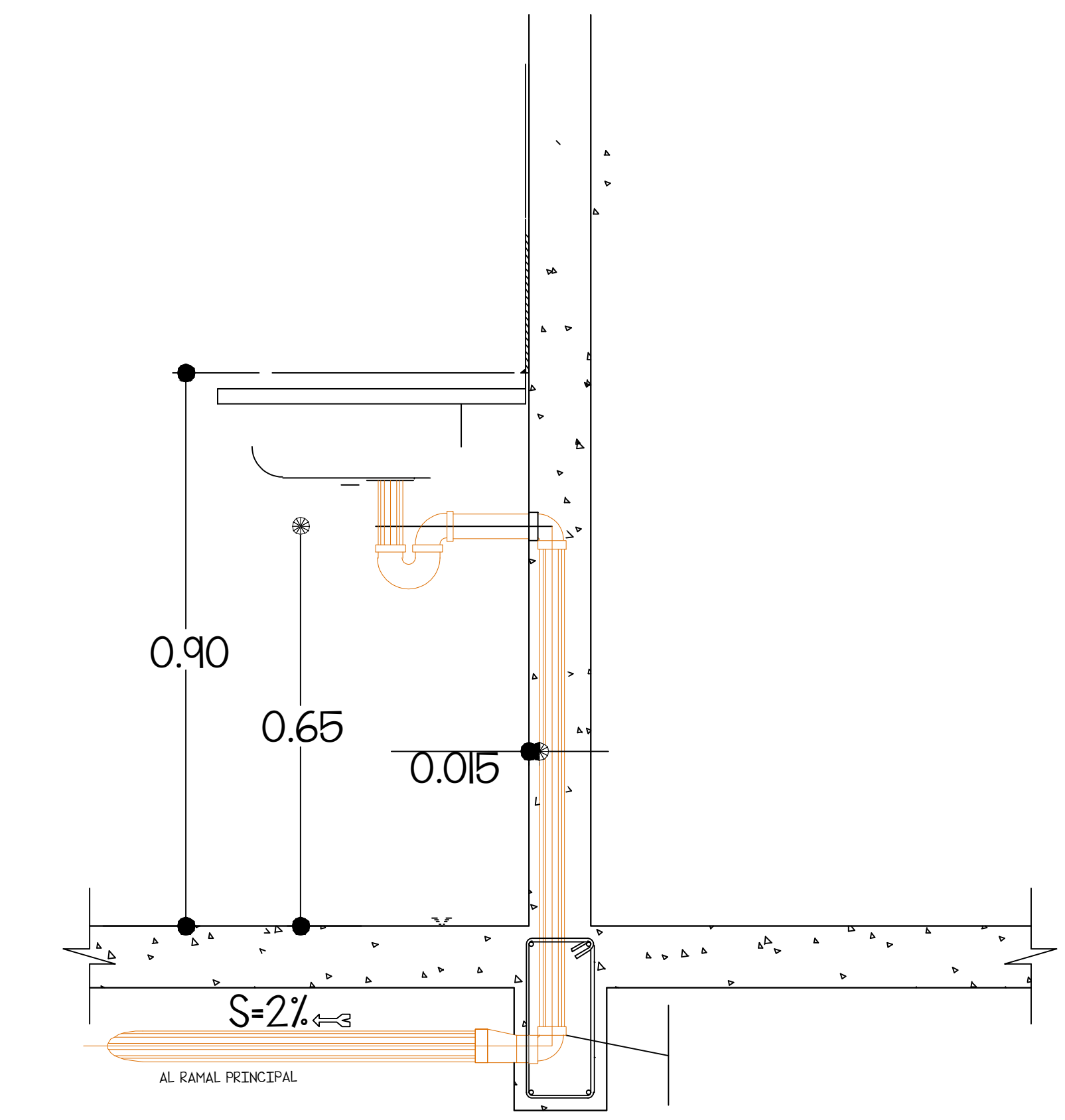
DESCARGA FREGADERO
