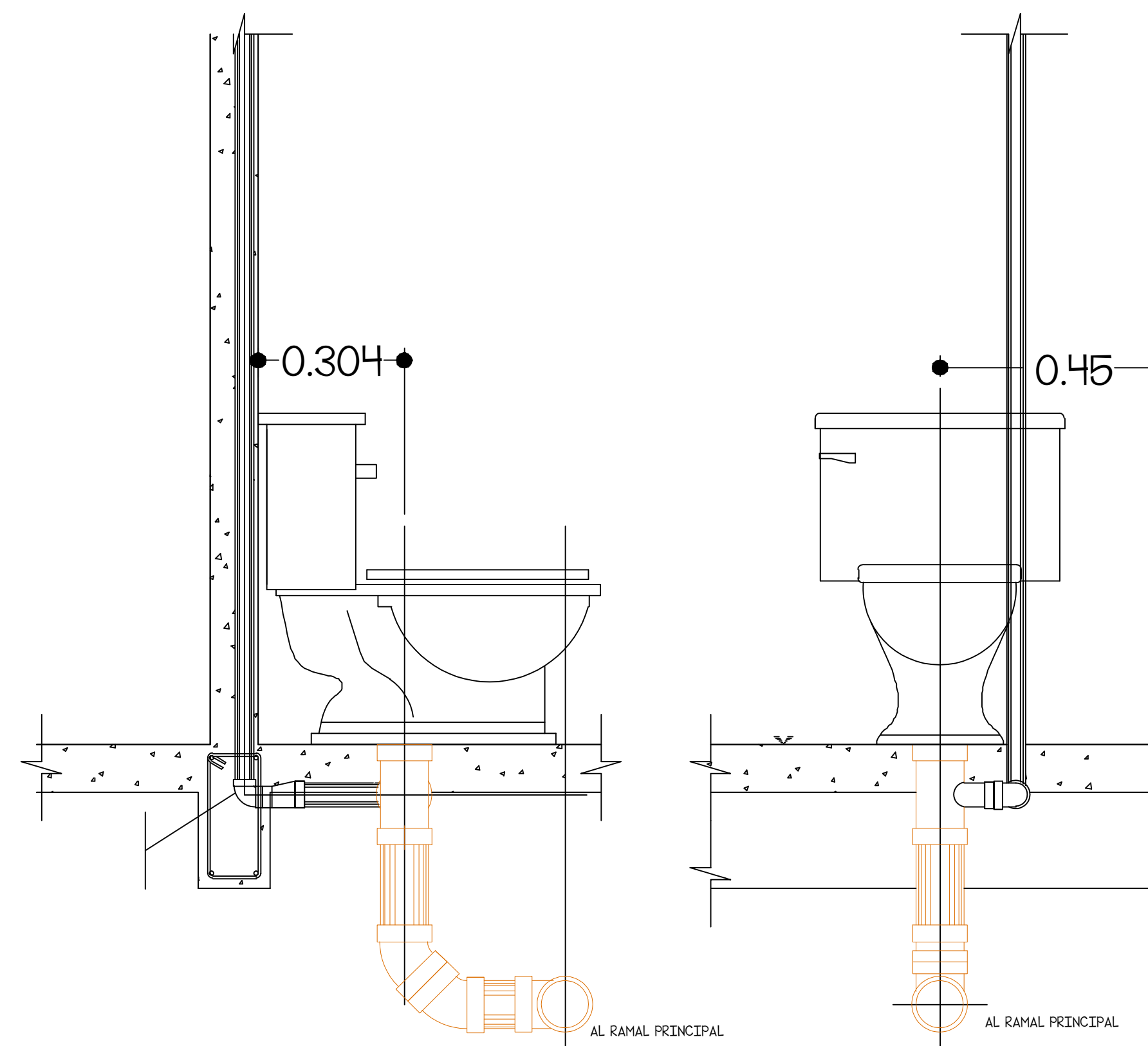
DESCARGA W.C
