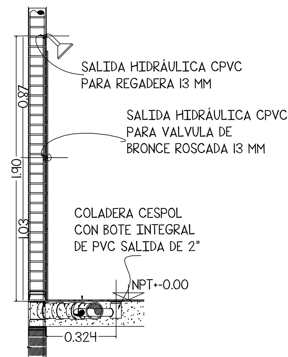
DETALLE DE REGADERA
