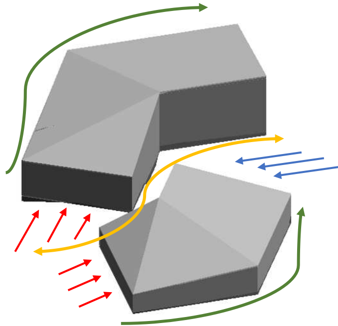
Imagen 22. Modelado Morfología
