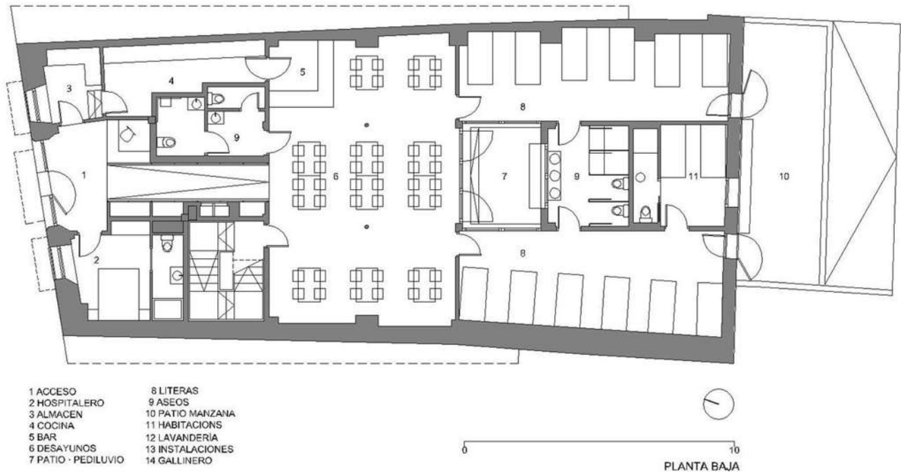
Imagen 4. Imagen de planta arquitectónica
