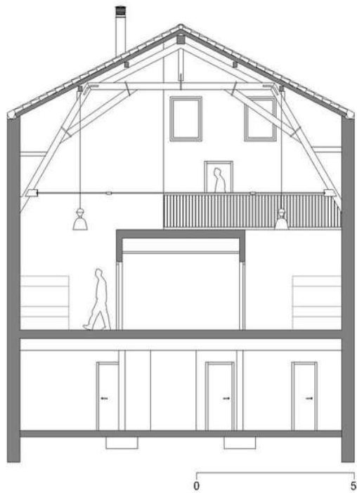
Imagen 7. Corte Arquitectónico del albergue
