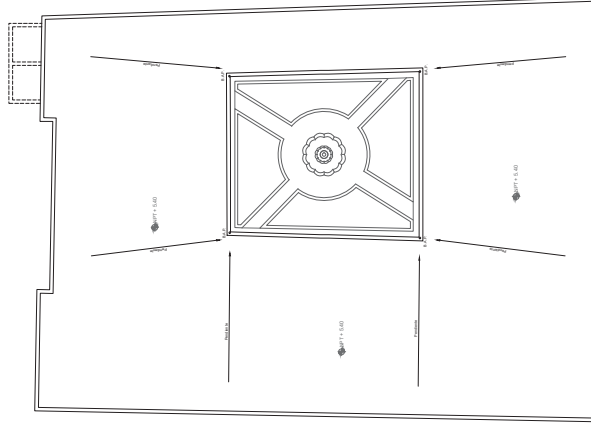
Planta de Conjunto Bajada de Agua Pluvial
