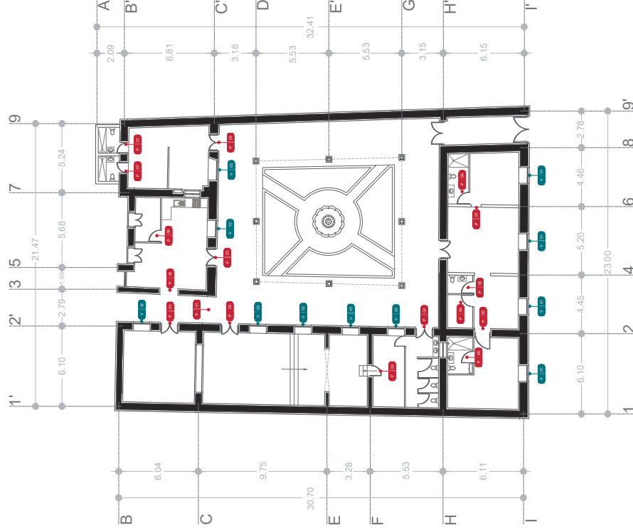
Planta de Carpintería
