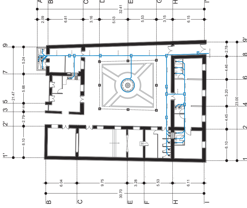
Planta de Instalación Sanitaria
