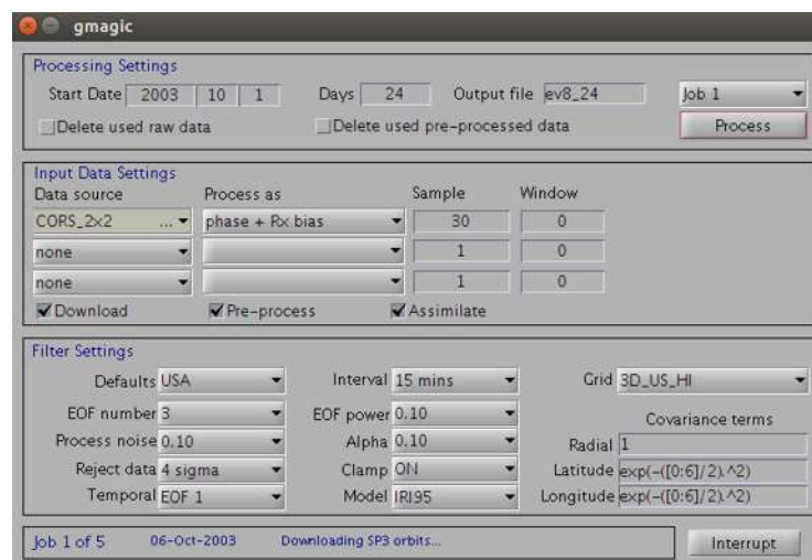
Figura 3.1: Interfaz gráfica del programa gmagic .
