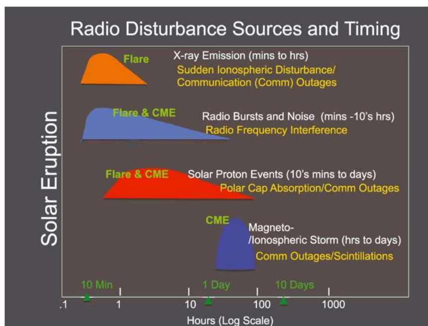
Figura 2.1: Tiempo aproximado de arribo (en escala logarítmica) para diferentes casos de actividad solar. Las letras blancas son los eventos solares, las amarillas son los efectos observables sobre la Tierra. Tomado de: Knipp et al., (2016)
