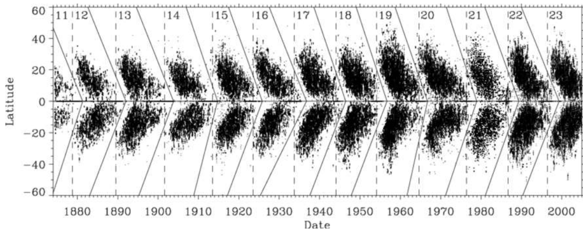
Figura 1.12: Distribución espacial de las manchas solares conocida como diagrama mariposa. Tomado de: Solanki et al., (2008)
