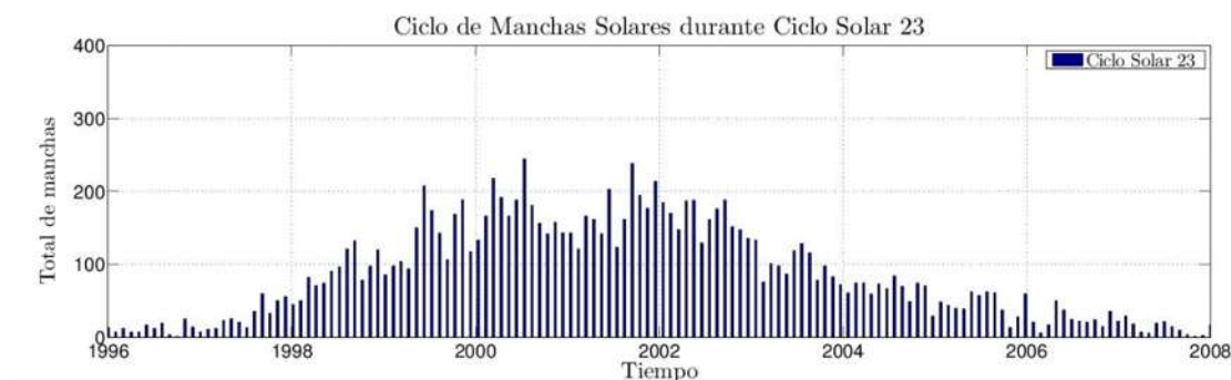
Figura 2.2: Manchas solares mensuales durante el Ciclo Solar 23 con datos obtenidos de SILSO data/image , Royal Observatory of Belgium, Brussels .
