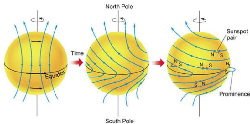
Figura 1.13: Descripción gráfica del movimiento de las manchas solares sobre la corteza. Tomado de: Pearson Prentice Hall, Inc. (2005).
