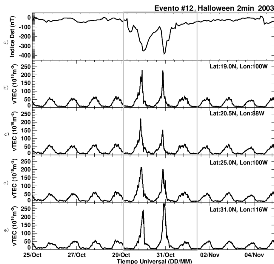
Figura 4.13: El panel a) indica el comportamiento del índice Dst en función del tiempo. Los cuatro paneles restantes (b), c), d) y e)) muestran el comportamiento del TEC vertical o vTEC con datos cada 2 minutos para el evento #12 a diferentes latitudes y longitudes (ver mapa 3.4) sobre territorio mexicano.
