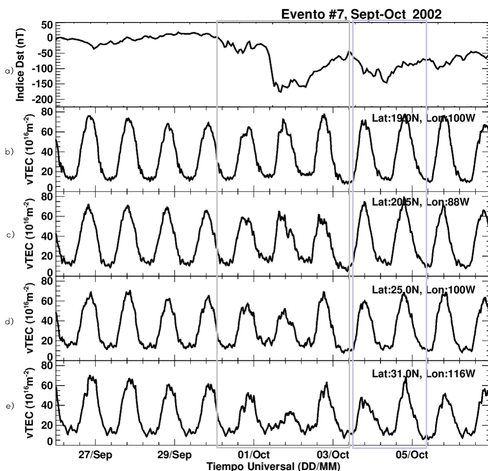
Figura 4.7: El panel a ) indica el comportamiento del índice Dst en función del tiempo. Los cuatro paneles restantes ( b ), c ), d ) y e )) muestran el comportamiento del TEC vertical o v\text{TEC} para el evento #7 a diferentes latitudes y longitudes (ver mapa 3.4) sobre territorio mexicano.
