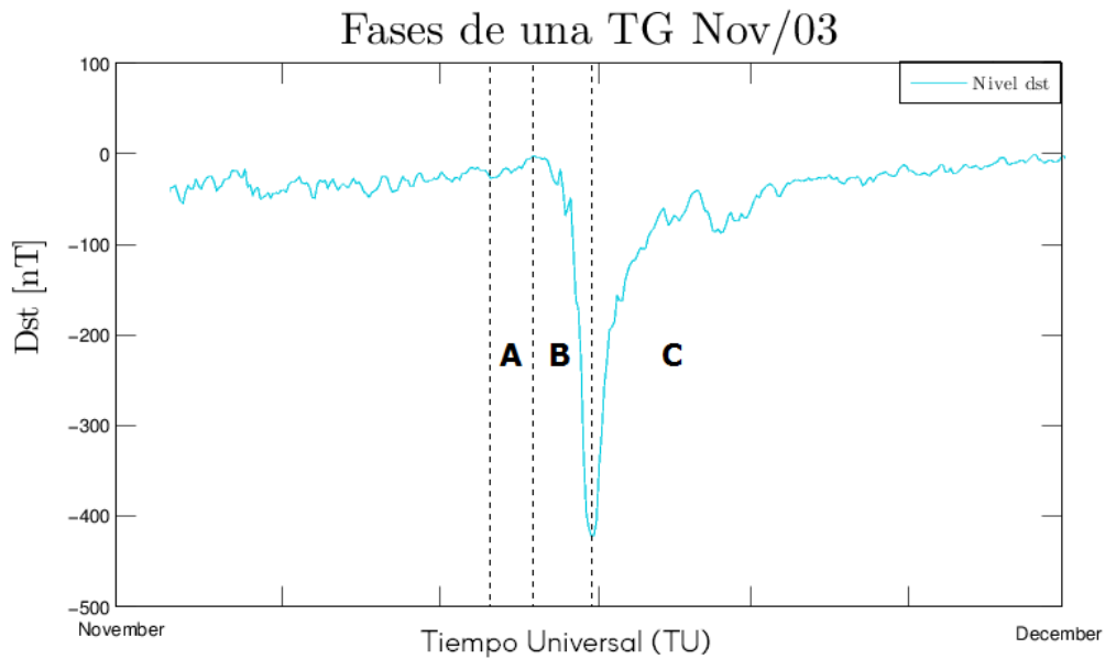
Figura 1.14: Gráfica de las tres diferentes fases de una tormenta geomagnética.
