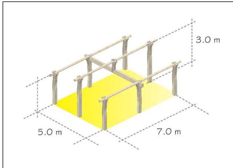
Figura 3-9. Dimensiones promedio de modulo base de vivienda de bajareque. Fuente: elaboración propia.
