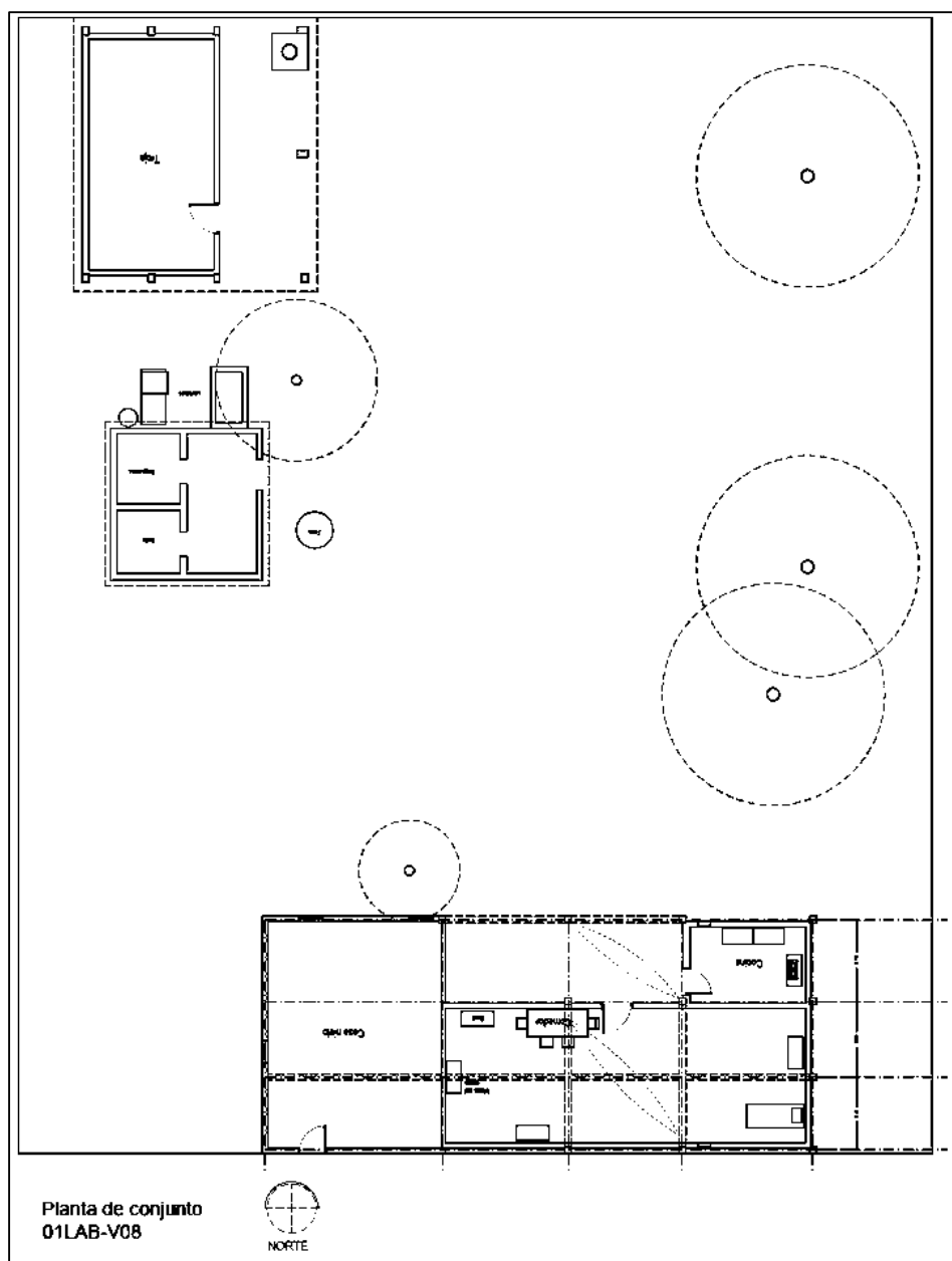
Figura 5-29. Planta de conjunto de vivienda en La Blanca. Clave:01LAB-V08. Fuente: elaboración propia.
