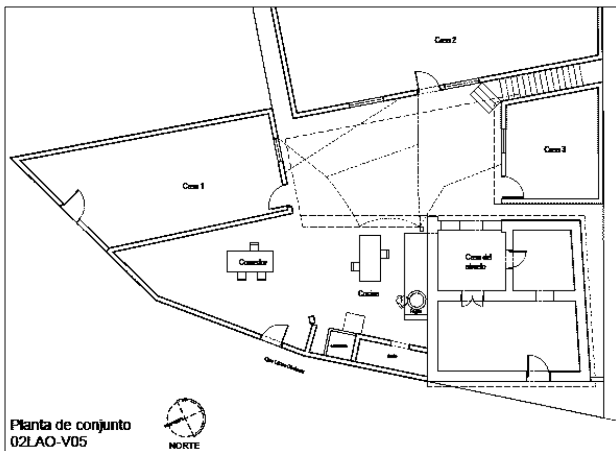
Figura 5-6. Planta de conjunto de vivienda en Laollaga. Clave:02LAO-V05. Fuente: elaboración propia.
