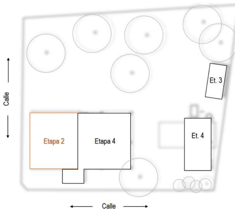
Figura 5-13. Sucesión constructiva, vivienda 02LAO-V04. Etapa 2: Vivienda de adobe de dos piezas; etapa 3: Baño y ducha de concreto; etapa 4: cocina y comedor adosado a la vivienda y cocina de leña separada de la vivienda. Fuente: elaboración propia.
