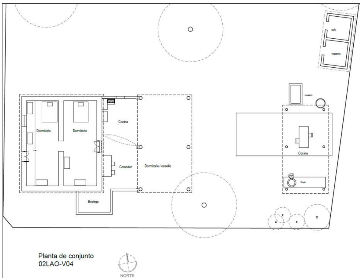
Figura 5-14. Planta arquitectónica de conjunto actual. Vivienda 02LAO-V04. Fuente: fotografía del autor, 2022.
