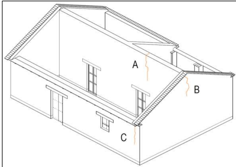
Figura 3-2. Principales grietas en muros de vivienda de adobe de Santiago Laollaga: A) muro central, B) muro piñón y C) esquina. Fuente: elaboración propia.
