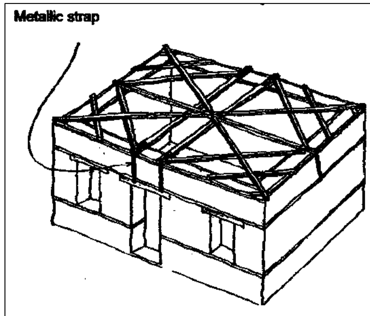
Figura 3-20. Ejemplo de solución para rigidizar entrepiso, utilizada en la isla griega de Galaxidi. Fuente: Touliatos, 2001. 37
