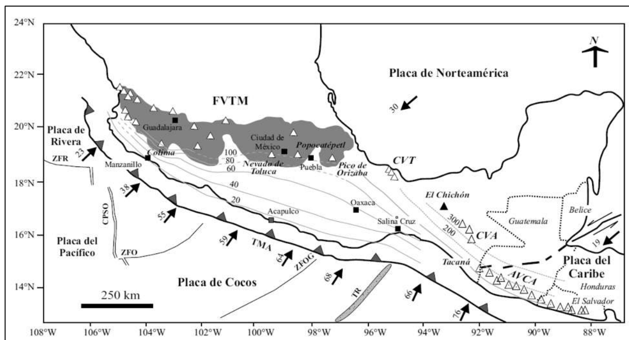
Figura 1-6. Distribución tectónica y volcánica del sur de México. FVTM refiere a la Faja Volcánica Transmexicana, CVT al Campo Volcánico de los Tuxtlas, CVA al Cinturón Volcánico de Chiapas y AVCA al Arco Volcánico de Centroamérica. Las líneas grises representan las curvas de igual profundidad de sismos. TMA: Trinchera Mesoamericana, ZFO: Zona de Fractura de Orozco, CPSO: Cresta Pacífica Oriental, ZFR: Zona de Fractura de Rivera, ZFOG: Zona de Fractura de O'Gorman, y TR: Ridge de Tehuantepec. Fuente: José Luis Macías, 2005. 86
