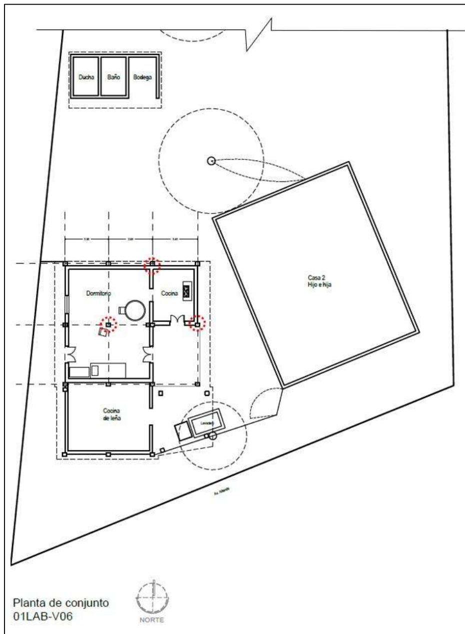
Figura 5-25. Planta de conjunto de vivienda 01LAB-V06. Círculos rojos representan horcones sustituidos por pilares de concreto. Fuente: elaboración propia.
