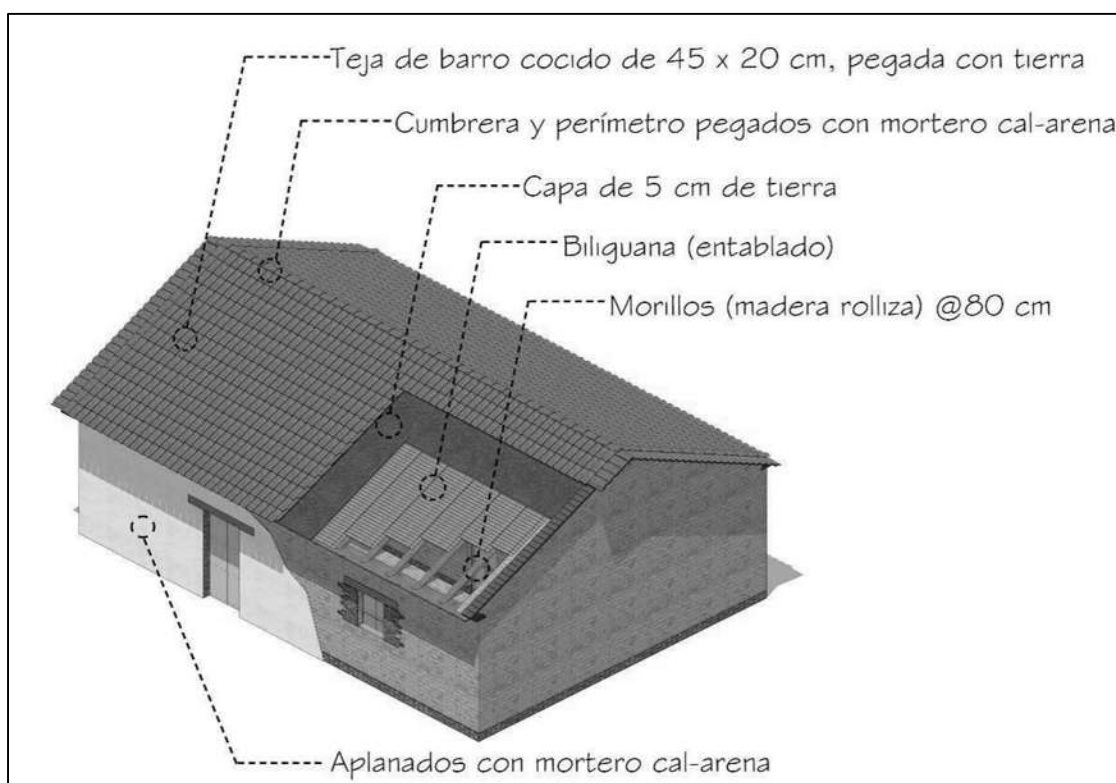
Figura 2-26. Proceso constructivo de la casa de adobe. Cubierta y acabados. Fuente: elaboración propia.
