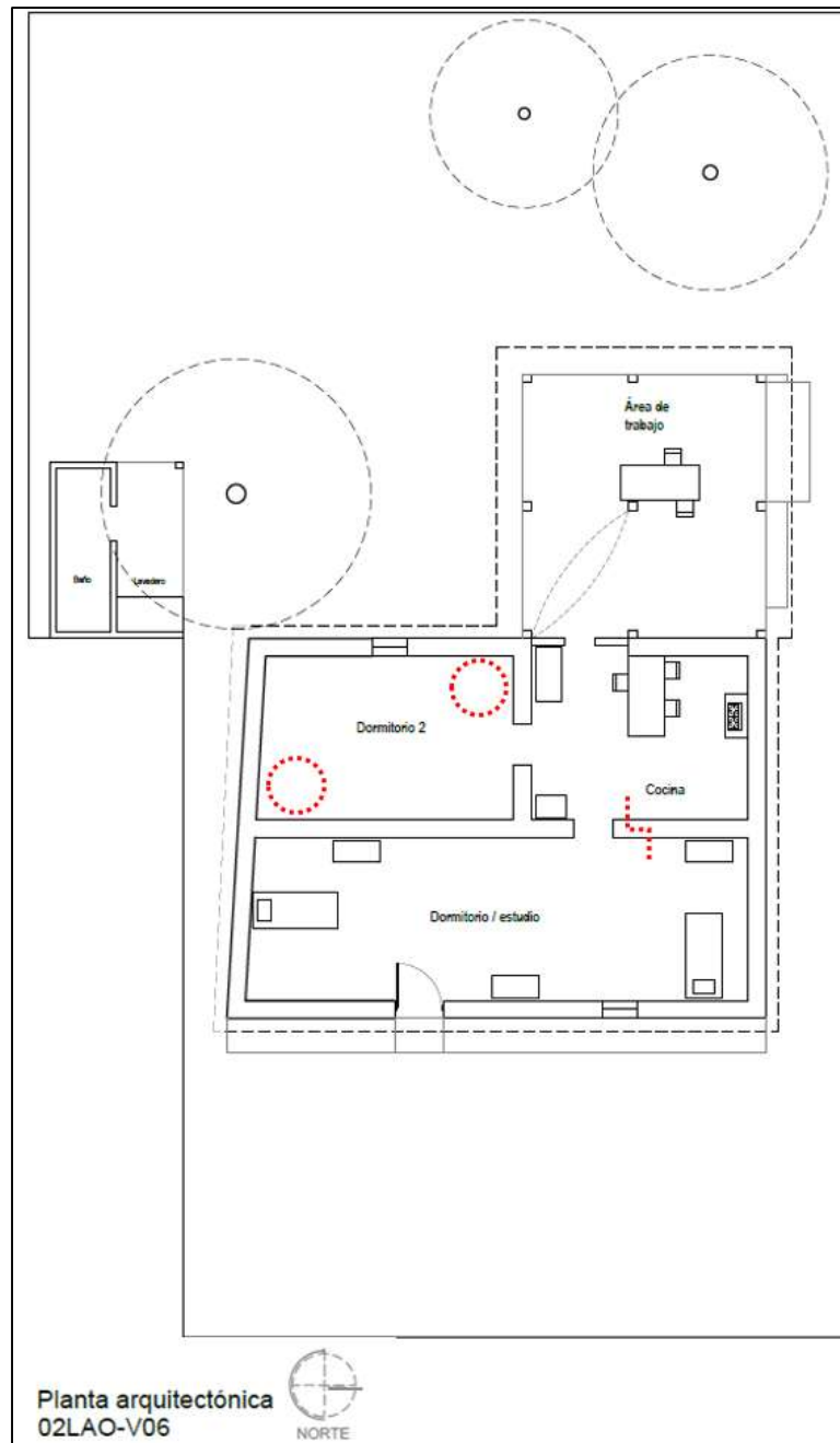
Figura 5-11. Planta arquitectónica. Estado actual, vivienda 02LAO-V06. Líneas punteadas en rojo representan agrietamientos. Círculos rojos refieren daños en cubiertas. Fuente: elaboración propia.
