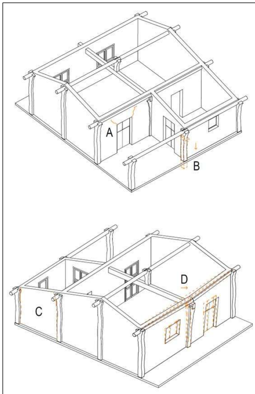
Figura 3-5. Daños mayores en la vivienda de bajareque de La Blanca, Sto. Domingo Ingenio: A) agrietamiento de vértices de puertas y ventanas B) hundimiento de pilares, C) Separación entre los muros y pilares y D) desplome de muros y pilares. Fuente: elaboración propia.
