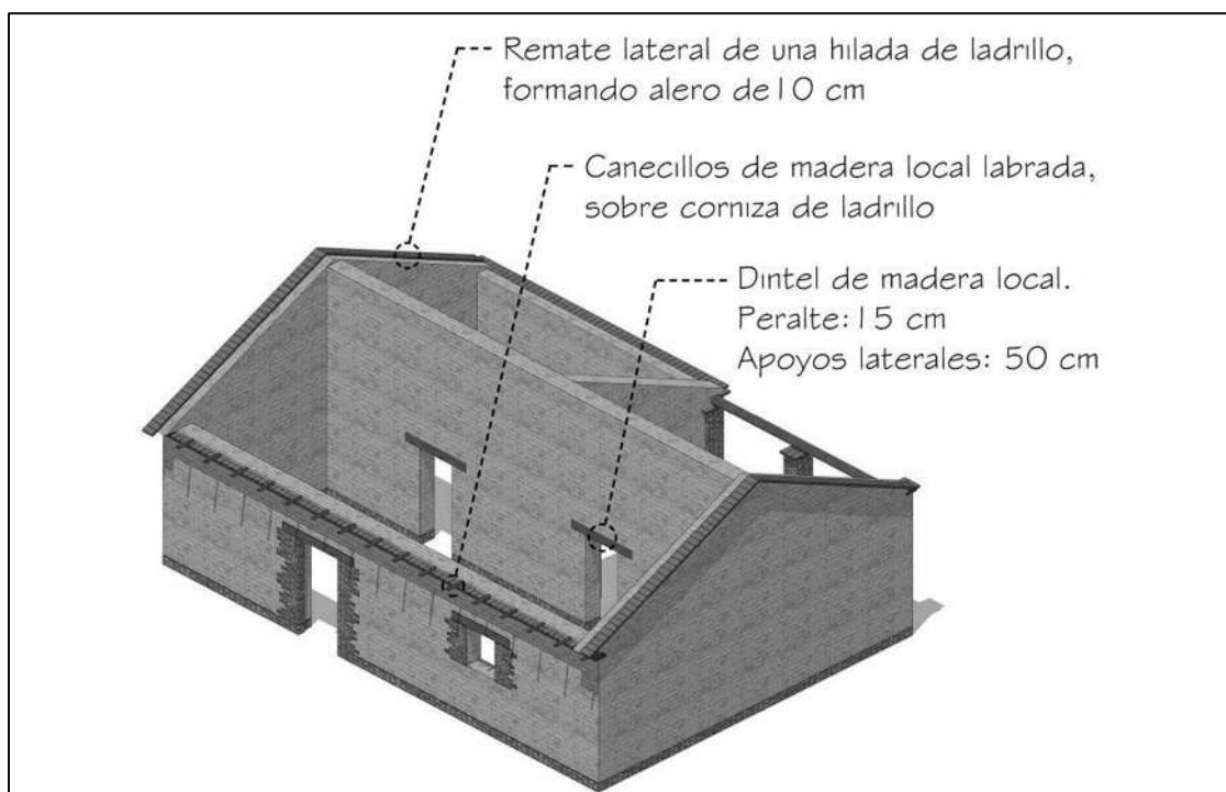
Figura 2-25. Proceso constructivo de la casa de adobe. Remate de muros, canecillos y dinteles. Fuente: elaboración propia.
