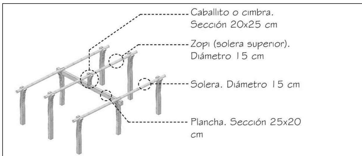
Figura 2-20. Procedimiento constructivo de la casa de barro: colocación de soleras, plancha y caballito. Fuente: elaboración propia.
