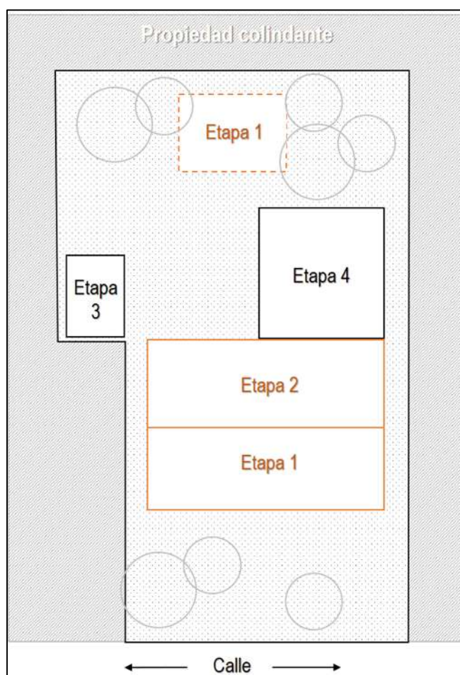
Figura 5-9. Sucesión constructiva, vivienda 02LAO-V06. Etapa 1: Crujía de adobe y palapa de palma; etapa 2: Recamara y corredor de adobe y cubierta de teja. Etapa 3: Módulo de baño, ducha y lavadero. Etapa 4: cubierta de concreto sobre pilares, para espacio de trabajo. Fuente: elaboración propia.
