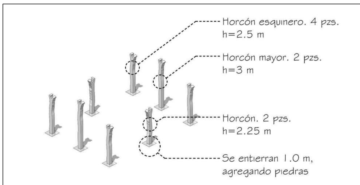
Figura 2-19. Procedimiento constructivo de la casa de barro: disposición de horcones. Fuente: elaboración propia.
