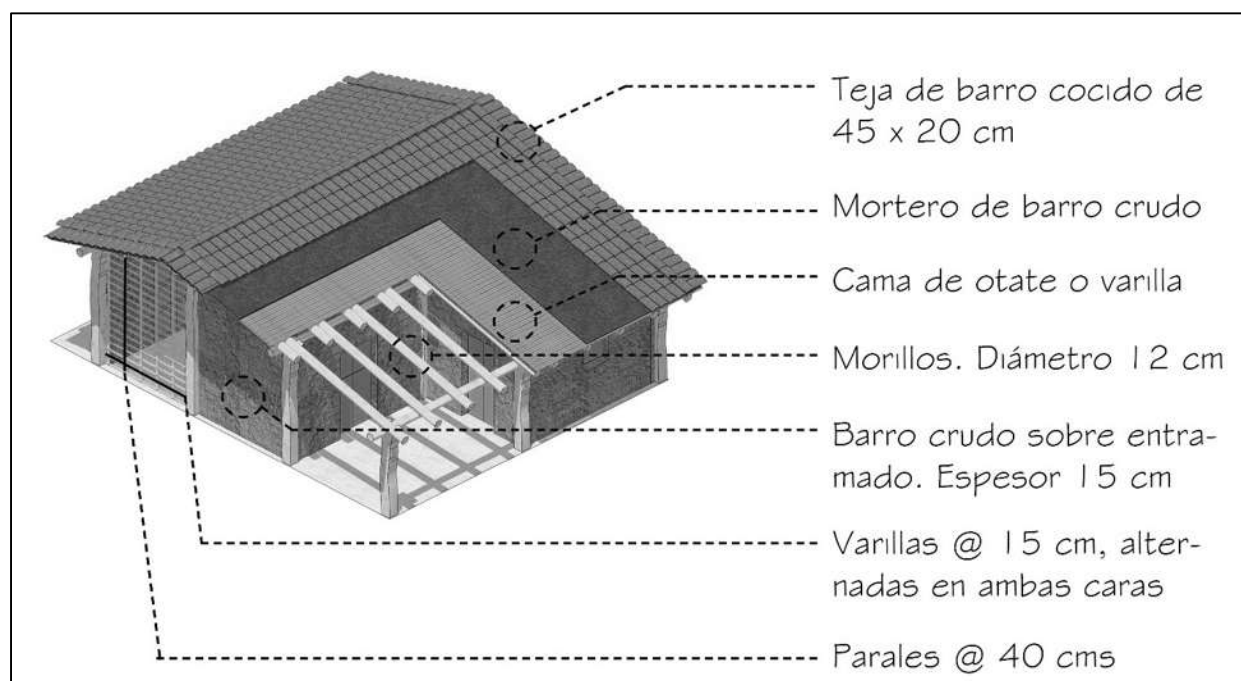
Figura 2-21. Procedimiento constructivo de la envolvente de la casa de barro. Fuente: elaboración propia.
