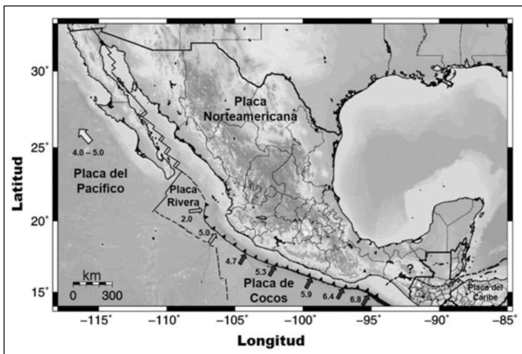
Figura 1-5. Interacción de placas tectónicas en el territorio mexicano. La dirección de movimiento se indica con las flechas. Los números indican la velocidad en cm/año. Fuente: L. Ávila Barrientos, 2021. 84
