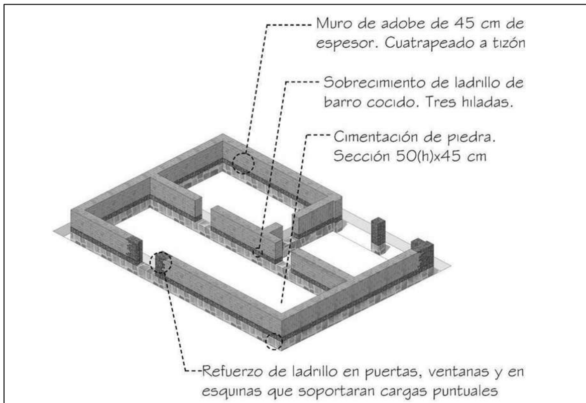
Figura 2-24. Proceso constructivo de la casa de adobe. Cimentación y desplante de muros. Fuente: elaboración propia.
