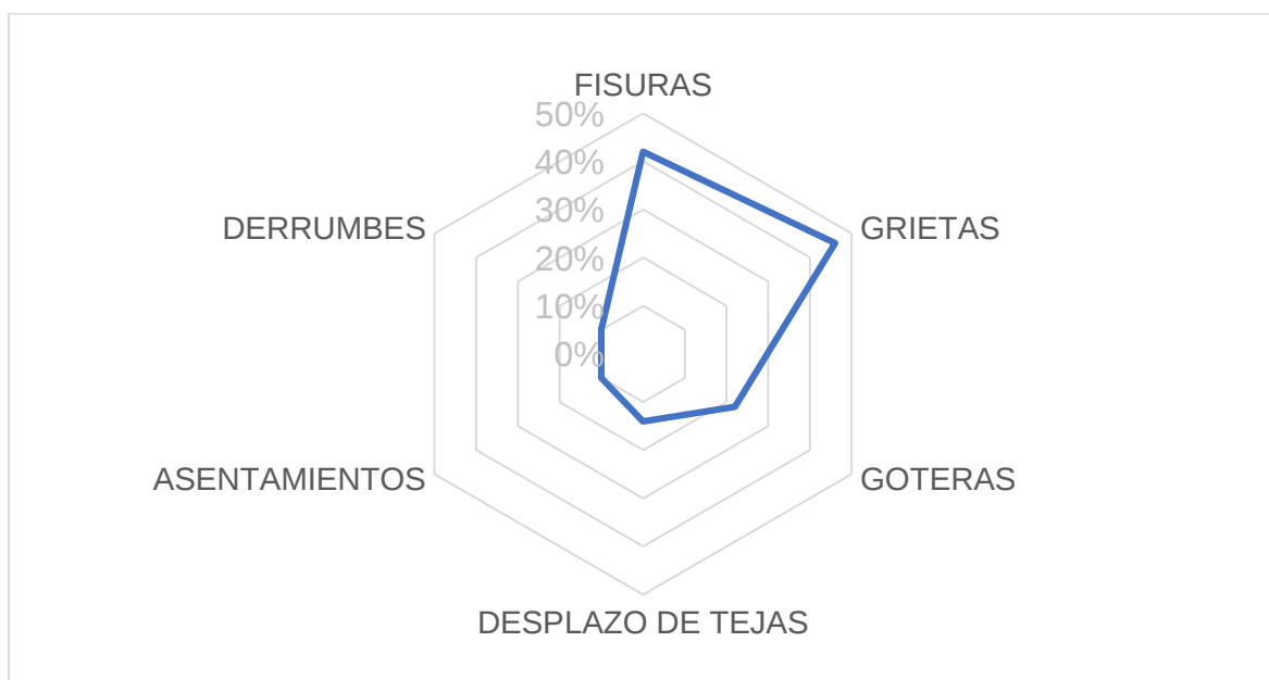
Figura 5-47. Tipos de daños por sismos en las viviendas. Fuente: elaboración propia.
