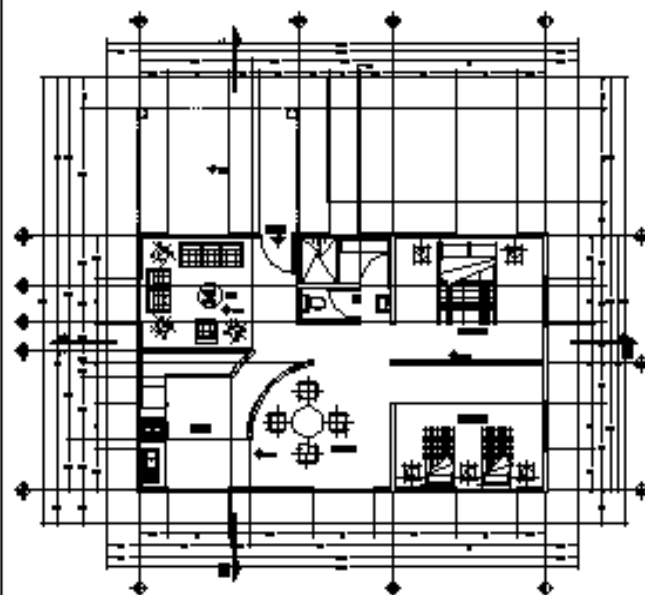
Casa 1 Planta Arquitectónica
