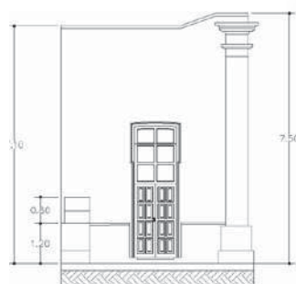
Fachada Sur
