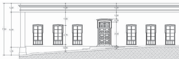
Fachada Este
