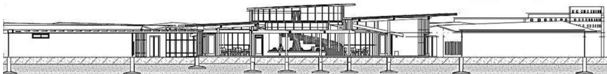
CORTE TRANSVERSAL-VISTA DEL VESTIBULO PRINCIPAL
